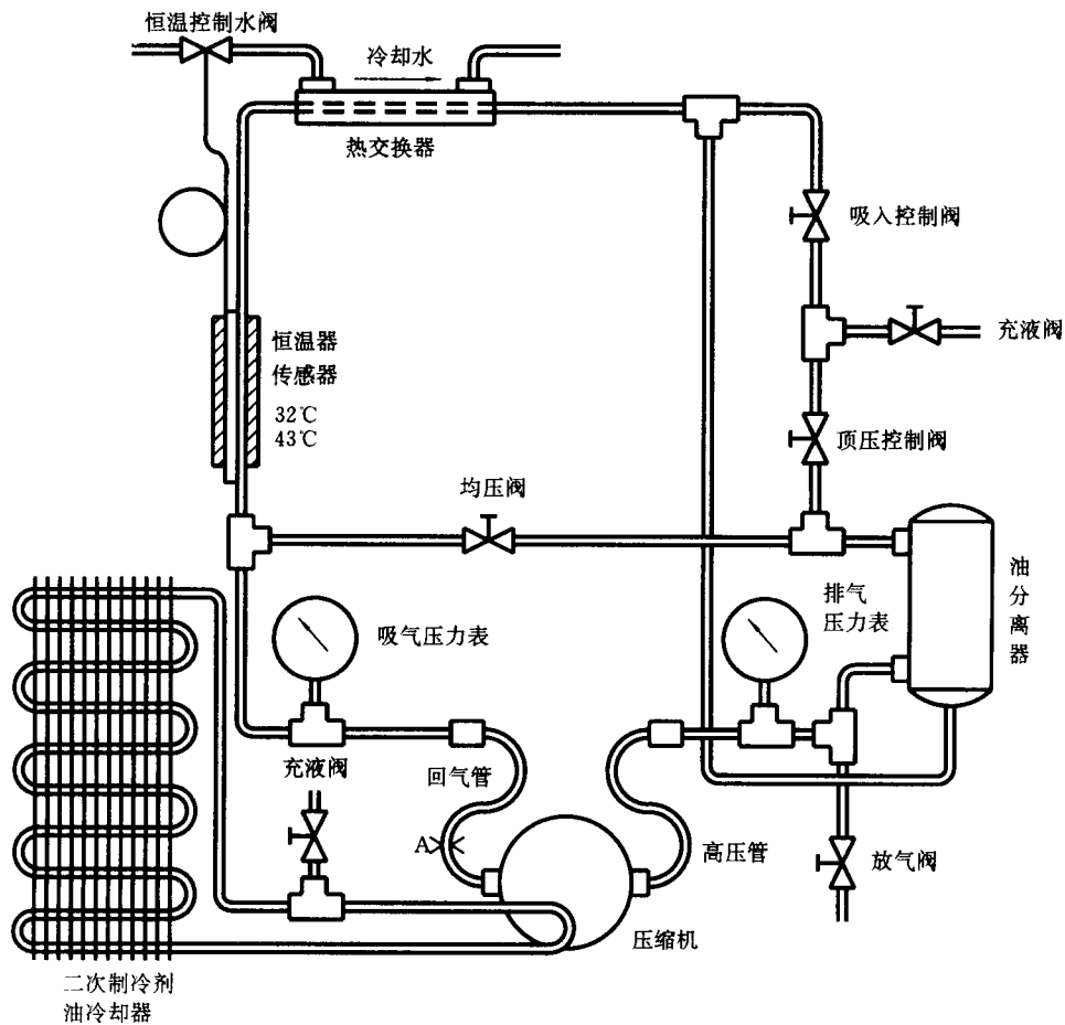
图 101 试验装置——代用冷却系统
