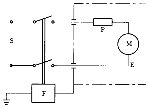
图 101 试验装置——代用冷却系统
