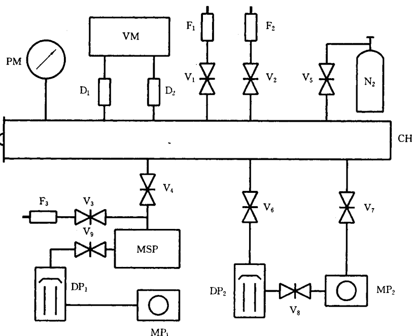
图 1 燃料棒氮质谱检漏系统示意图
