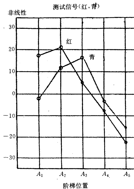
图 6.2.7.2 色度信号非线性失真举例
