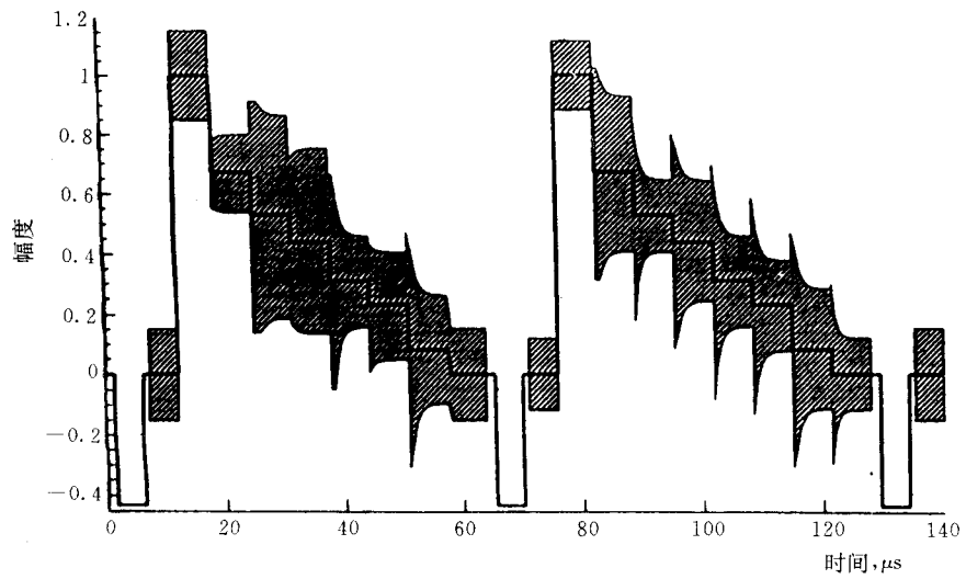
图 3.2.1.2(f) SECAM 彩条信号(100/0/75/0)
