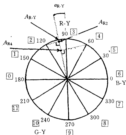
图 B1 R-Y 色差信号的相位角
