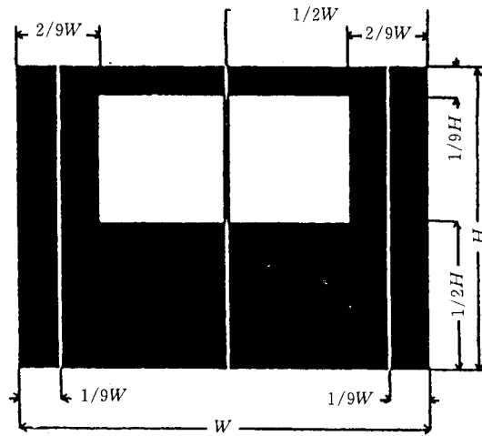
图 3.2.1.8 线条和窗口信号
