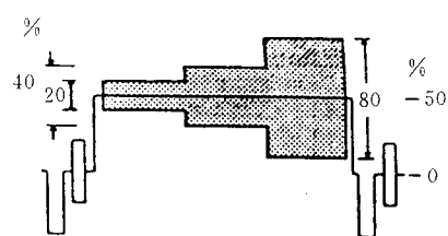
图 3.2.1.24 已调基座信号
