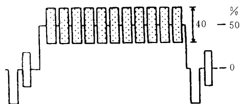
图 3.2.1.26 偏离载波的彩条信号
