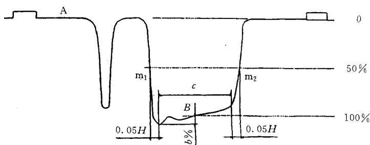
图 6.2.5.1 调制 2T 条响应
