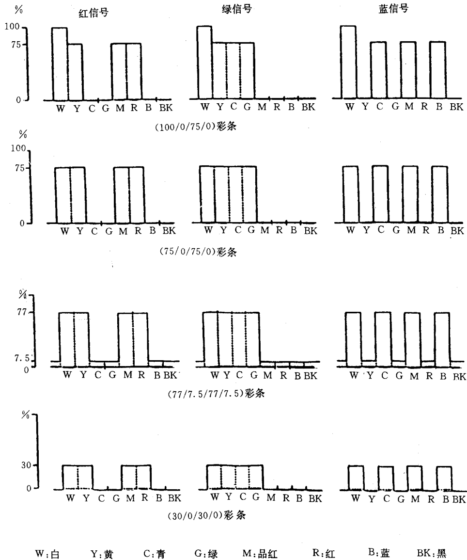
图 3.2.1.1 基色彩条信号
