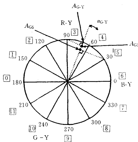
图 B2 G-Y 色差信号的相位角
