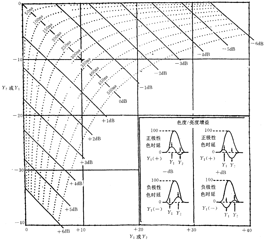
图 6.2.12.2 M/NTSC 制调制 20T 列线图 ( T=0.125 \mu s )
