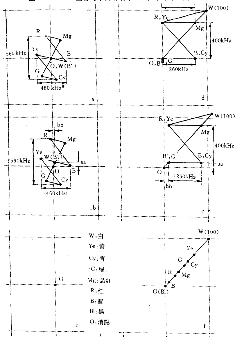
R-Y, B-Y 色差信号 RGB 基色信号 图 6.3.6.1 R-Y/B-Y 色差信号显示 a, b, c; R/B 基色显示 d, e, f (没有频率偏离误差: a 和 d; 有频率误差: b 和 e; 零饱和度: c 和 f)
