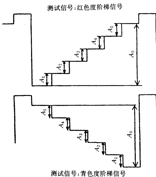
图 6.2.7.1 输出信号波形
