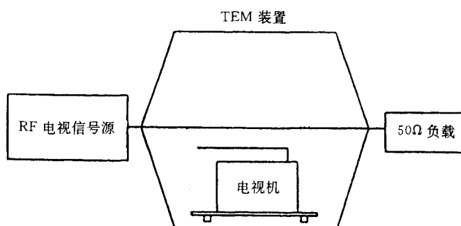
图 3.4.3.2 TEM 装置法的设备布置
