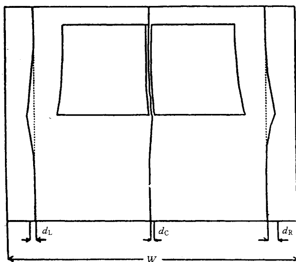
图 7.3.2.1 局部图像失真的测量
