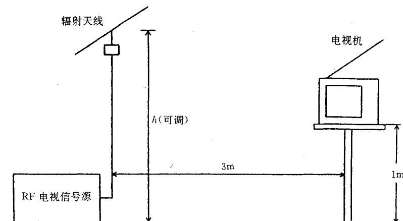
图 3.4.3.1 辐射天线法的设备布置
