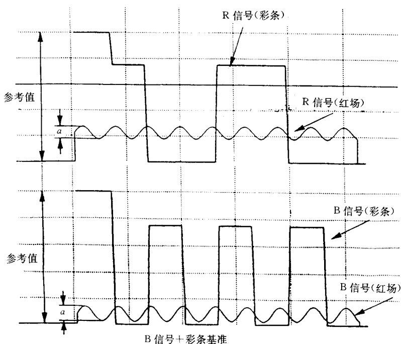
图 6.3.8.1 在 SECAM 制 R 和 B 信号中由于色串扰引起的差拍干扰
