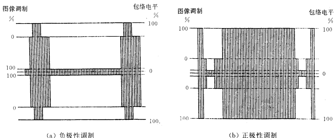
图 3.3.1 已调射频信号
