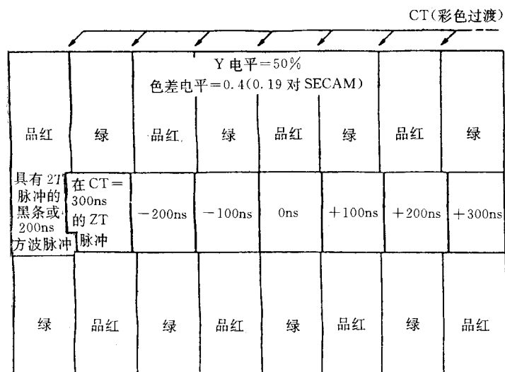
(a) Y/C 定时测试图
