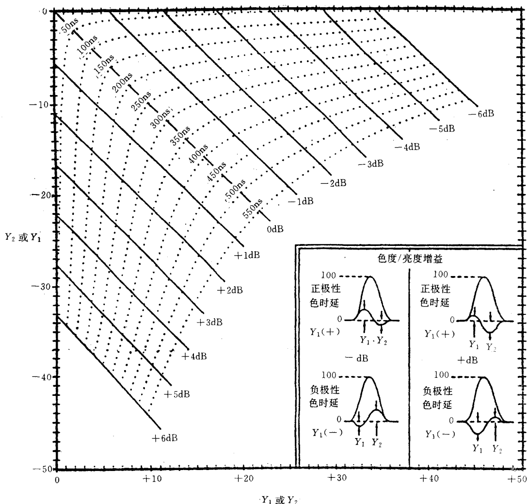
图 6.2.12.3 B, G/PAL 制调制 20T 列线图 ( T=0.100 \mu\text{s} )
