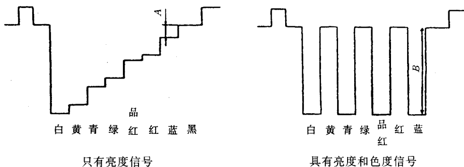
图 6.2.2.1 B 基色信号波形
