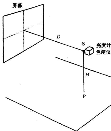
S: 标准观察位置; D: 标准观察距离; H: 标准观察高度; P: S 的投影点
