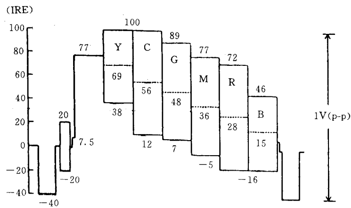
图 3.2.1.2(c) NTSC 彩条信号(77/7.5/77/7.5)
