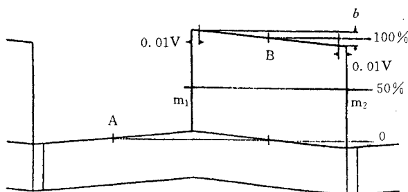
图 6.1.4.3 场频方波响应
