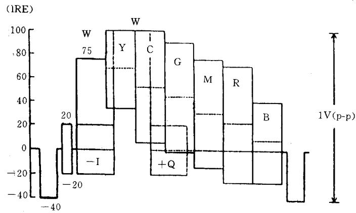
图 3.2.1.2(b) NTSC 彩条信号(75/0/75/0)
