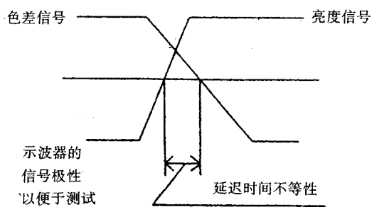
图 6.2.6.1 亮度/色度时延
