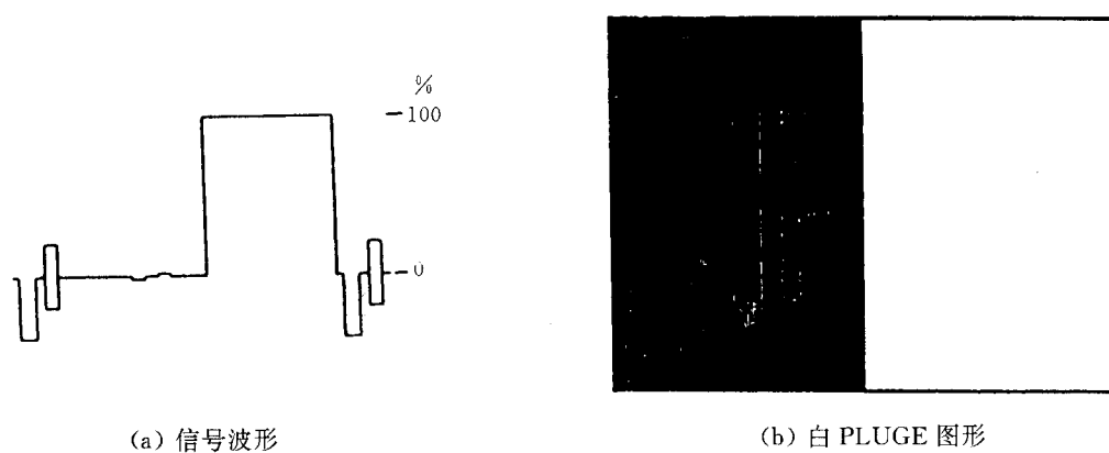
图 3.2.1.18 白 PLUGE 信号
