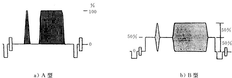
图 3.2.1.21 调制 20T 脉冲和条信号
