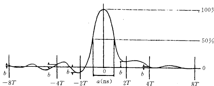
图 6.1.4.2 2T 脉冲响应
