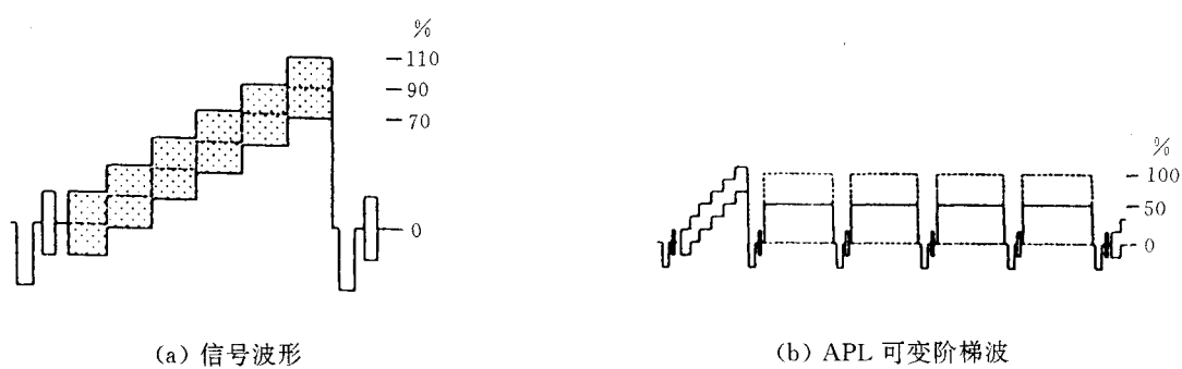
图 3.2.1.19 彩色阶梯信号
