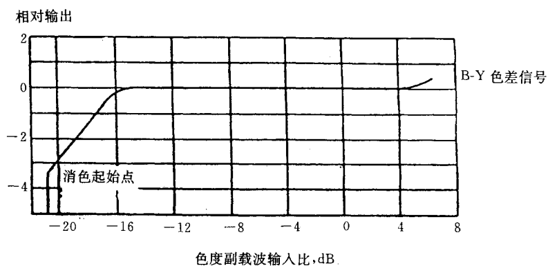
图 6.2.2.2 色度自动控制特性举例
