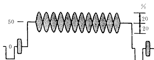
图 3.2.1.20 正弦波调制色度信号
