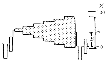
图 3.2.1.23 色度信号调制的阶梯波信号
