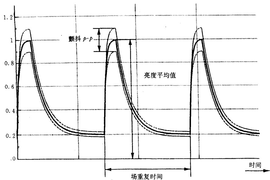
图 7.1.10.1 用异步电源工作对屏幕光输出特性影响的举例
