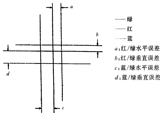
图 7.1.7.2 在交叉点处会聚和重合误差的测量
