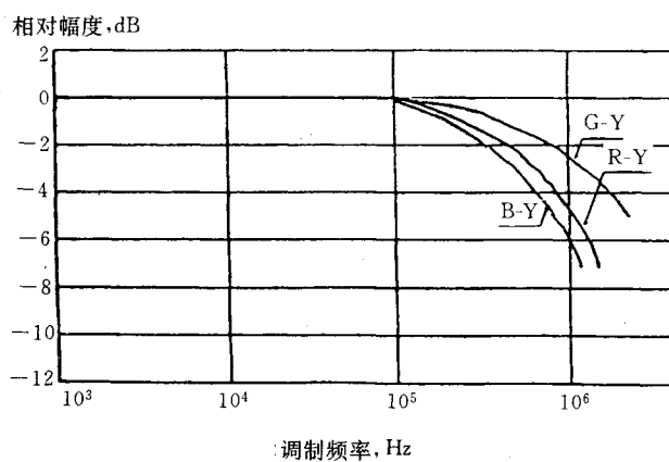
图 6.2.4.1 色度输出信号幅度对调制频率响应举例
