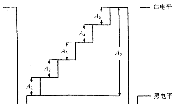
图 6.1.4.4 行期间非线性失真
