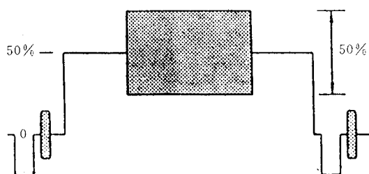
图 3.2.1.25 单彩条信号
