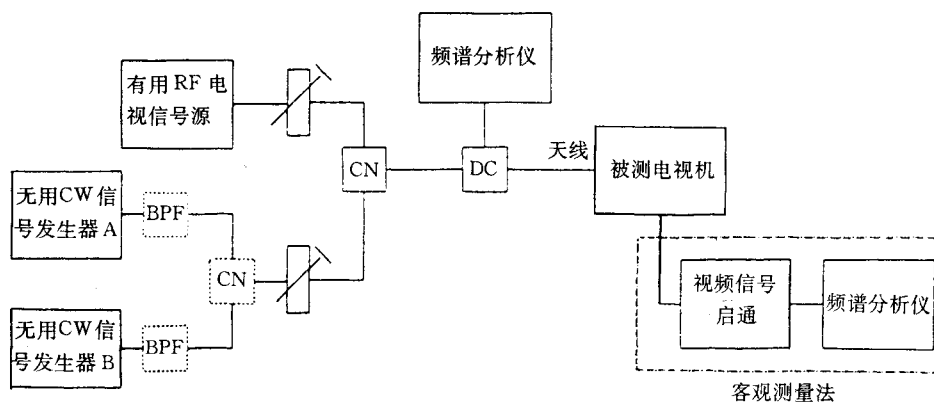
图 5.3.1.1 两信号法测试设备的连接
