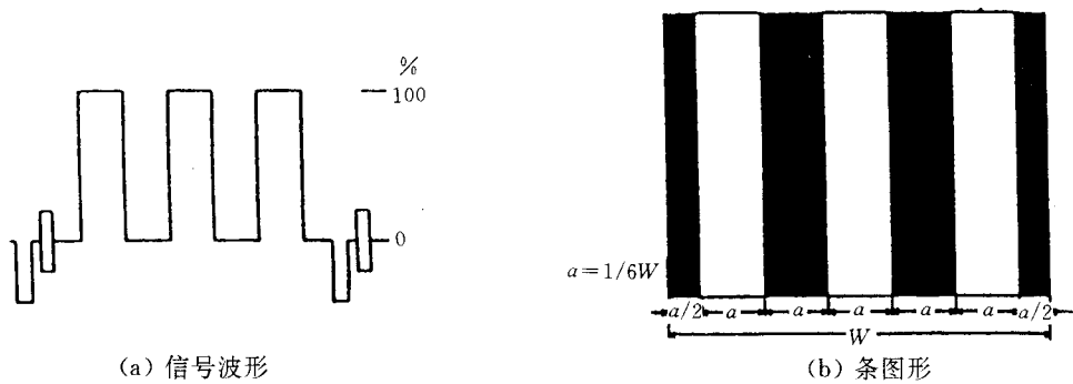
图 3.2.1.3 三垂直条信号
