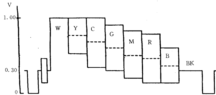
图 3.2.1.2(e) PAL 彩条系信号(100/0/75/0)
