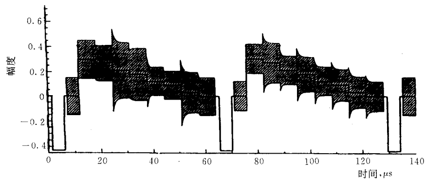
图 3.2.1.2(g) SECAM 彩条信号(30/0/30/0)
