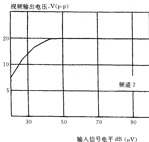
图 5.2.7.1 AGC 控制特性举例
