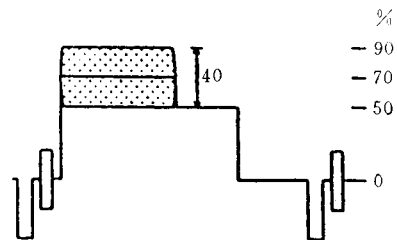
图 3.2.1.10 彩色基准信号
