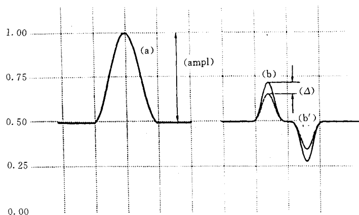
左:有正常色同步相位的蓝输出端 右:色同步相位 90°的蓝输出端 图 6.3.3.1 图像小面积失真,百叶窗的峰-峰值
