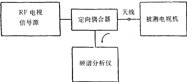
图 5.1.1.1 测量本振频率的设备连接
