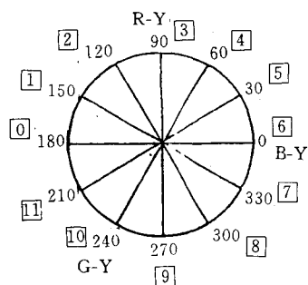
图 6.3.1.1 偏离载波彩条信号的矢量图
