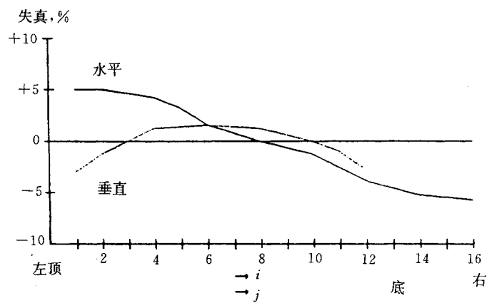
图 7.1.2.2 非线性图形失真举例
