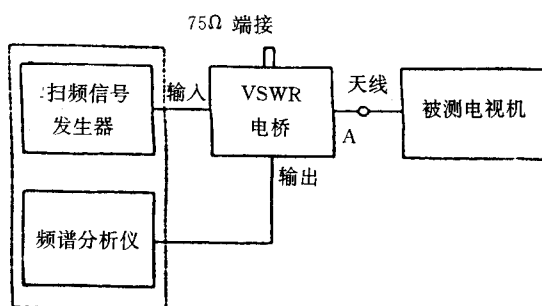
图 5.2.6.1 回波损耗测试仪器的连接
