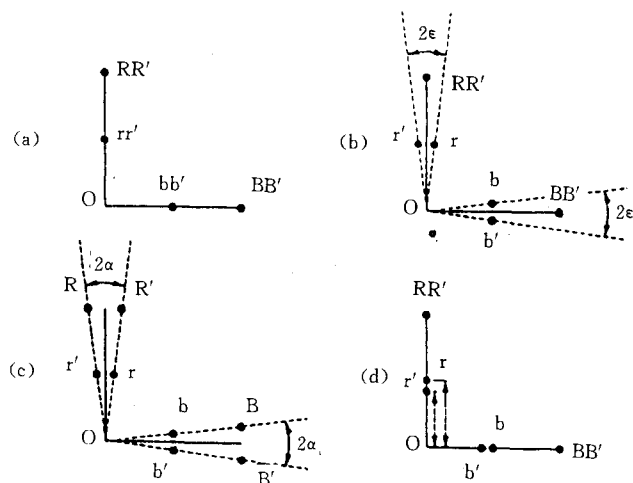
图 6.3.2.1 解调四行色差信号的矢量 X-Y 的表示
