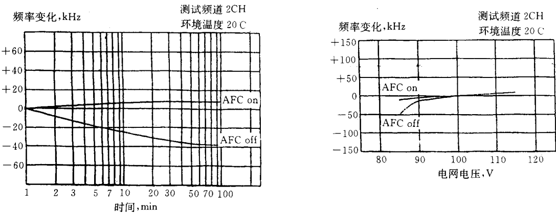
图 5.1.1.2 工作频率稳定度举例
