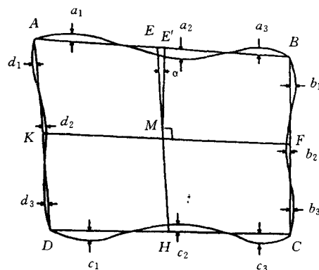
图 7.1.2.3(a) 测量轮廓失真的点
