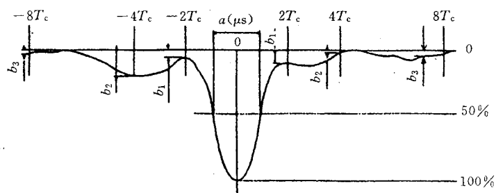
图 6.2.5.2 调制 20T 脉冲响应
