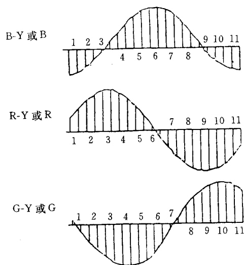
图 6.3.1.2 行扫描期间彩色输出信号波形
