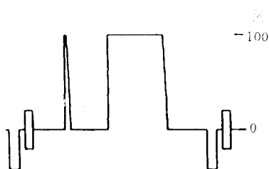
图 3.2.1.14 2T 脉冲和条信号
