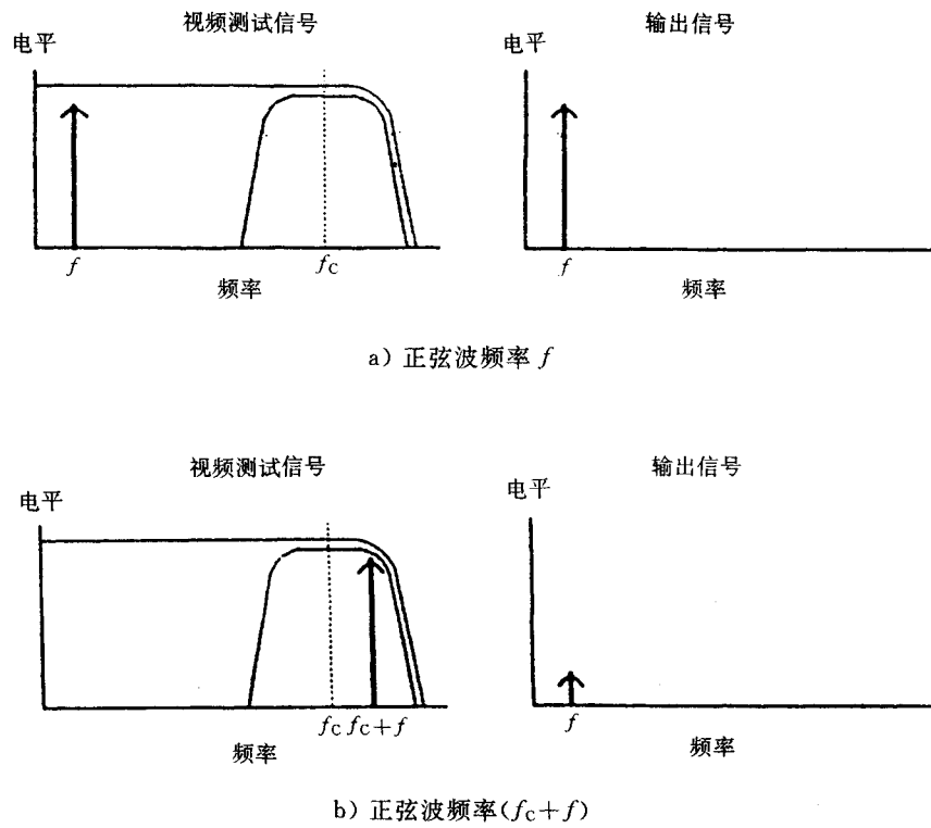
图 6.2.11.2 串色失真信号的频测试信号和输出信号的频率和电平
