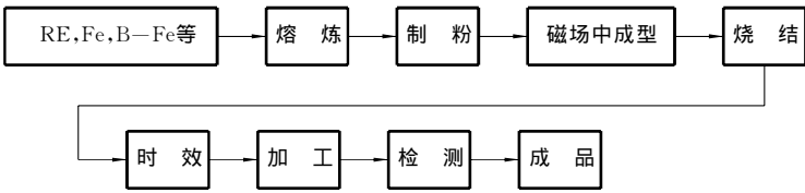
图 C1 烧结钕铁硼永磁材料工艺流程
