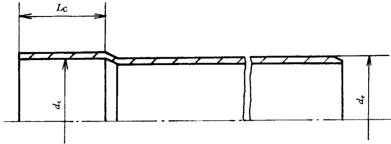
图 3 溶剂粘接型承插口
