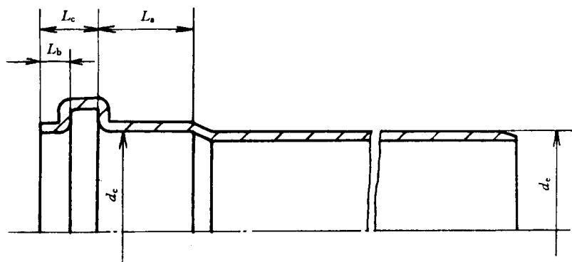
图 4 弹性密封连接型承插口
