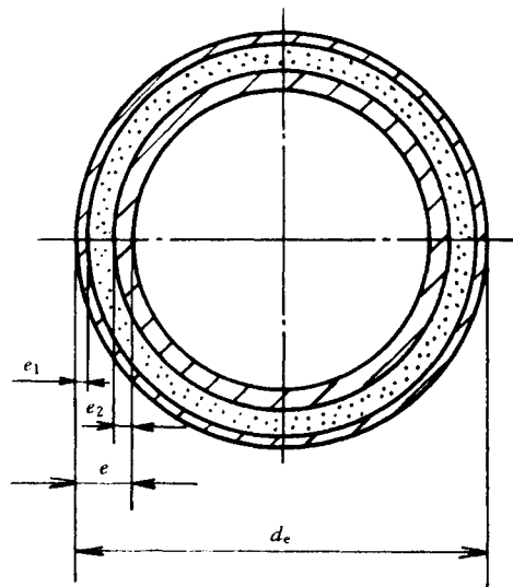
图 1 管材截面尺寸
