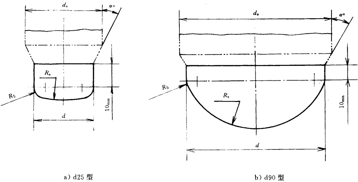
图 A1 冲头形状 表 A1 冲头尺寸
