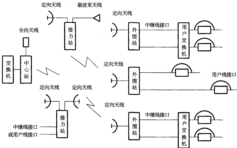
图 1 中继线型点对多点通信系统示意图
