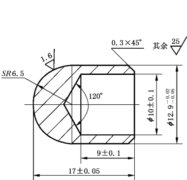
图 A1 试验弹丸
