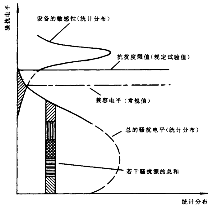
图 2 计及统计特性,电磁骚扰不同电平之间的关系
