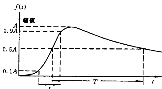
图 B2a) 单向浪涌
