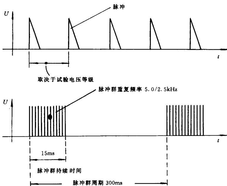
图 A12 快速瞬变概略图
