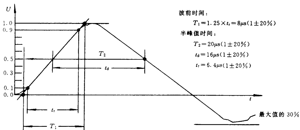
图 A8 开路电压波形
