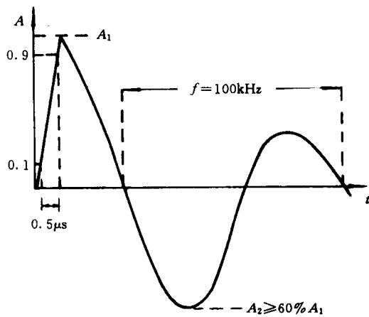
图 A14 振铃波特性(开路电压)
