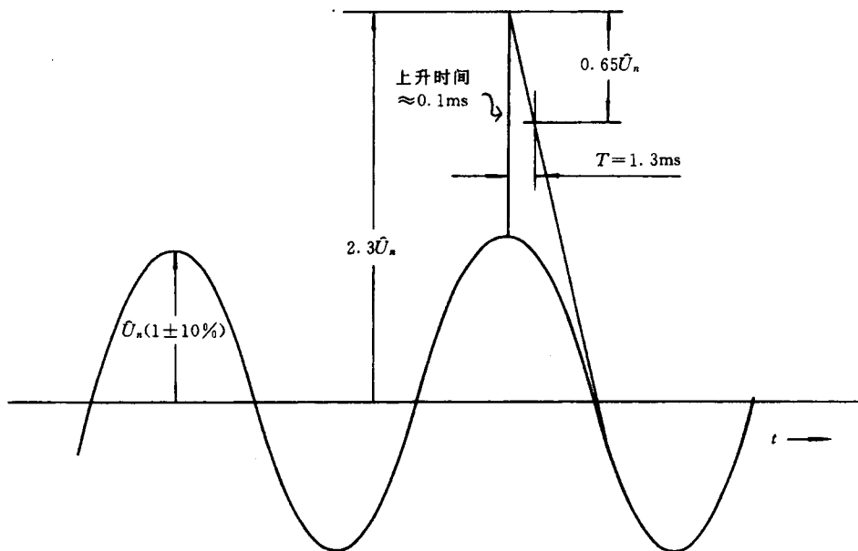
图 A7 典型长持续时间脉冲的波形
