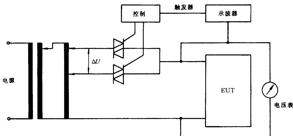
图 A5 发生器简图
