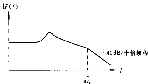
图 B2d) 振荡浪涌幅密度图的包络线
