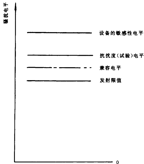
图 1 电磁骚扰不同电平之间的关系
