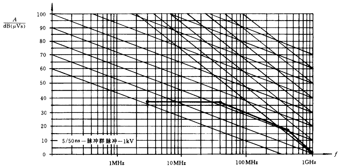
图 B5 试验瞬态的幅密度频谱
