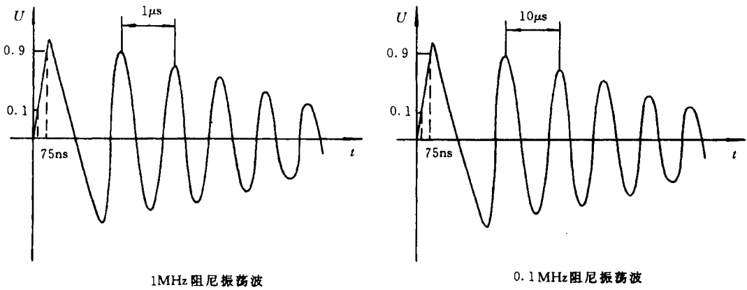
图 A16 阻尼振荡波特性
