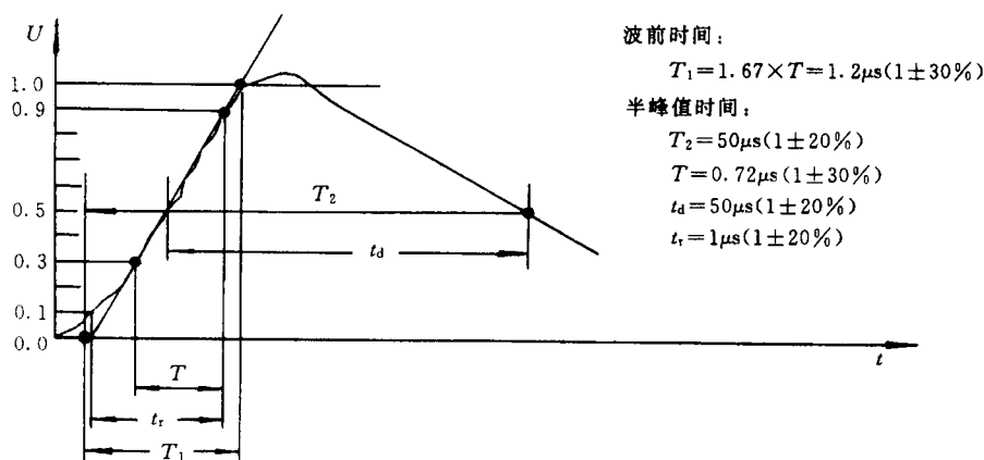
图 A8 开路电压波形
