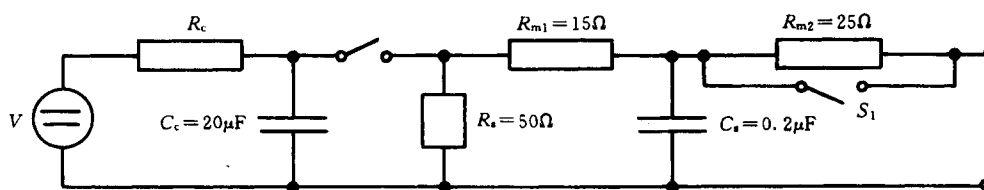
图 A18 试验发生器简图
