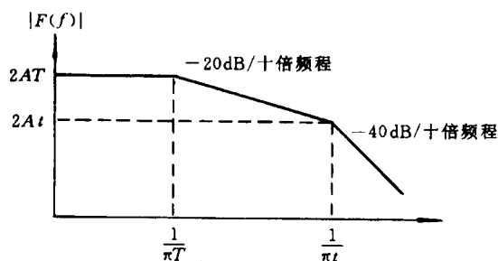
图 B2c) 单向浪涌幅密度图的包络线
