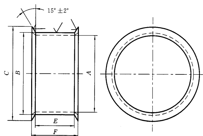
图 2 AL-1 双缘丝轴
