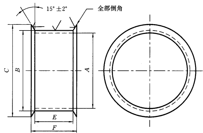
图 4 AL-3 双缘加宽丝轴
