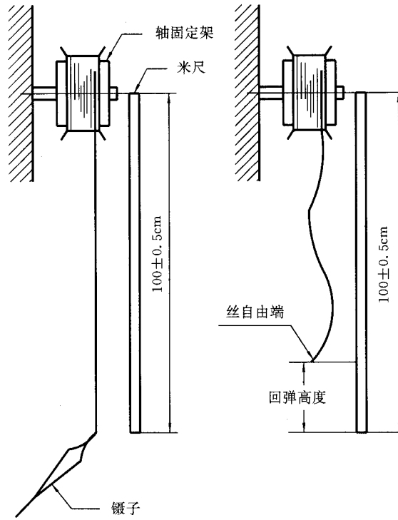
图 A1 金丝卷曲试验装置示意图
