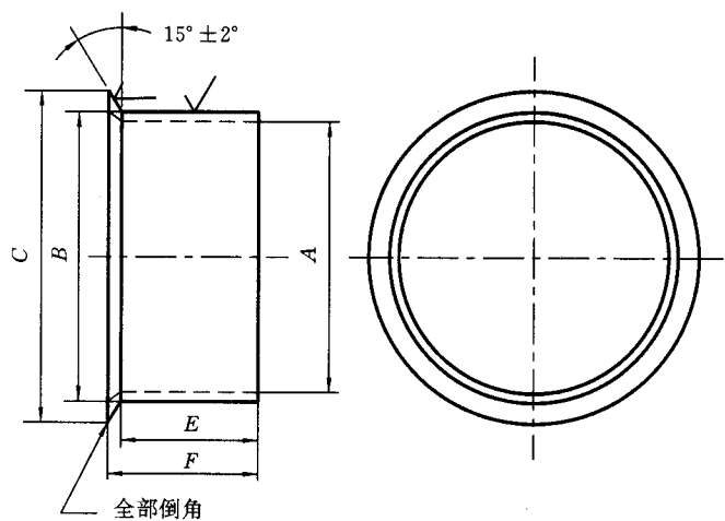
图 5 单缘加宽丝轴
