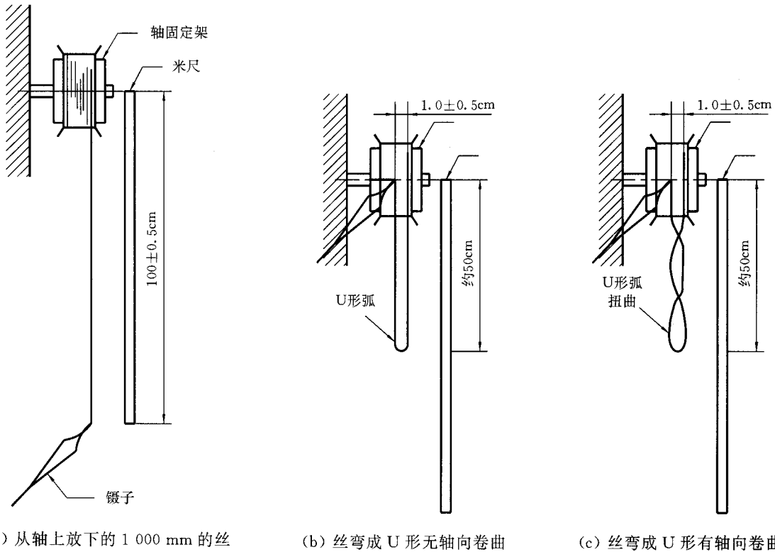
图 A2 金丝轴向扭曲试验装置图
