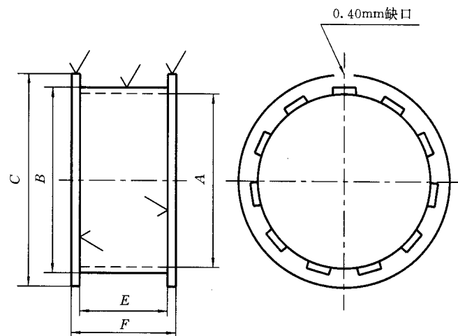
图 1 AL-0 丝轴
