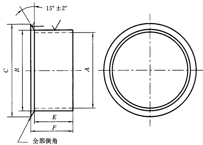
图 3 AL-2 单缘丝轴
