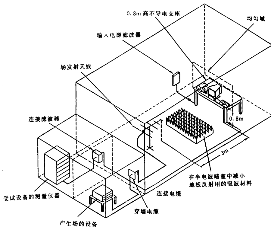
图 2 典型的试验设施举例
