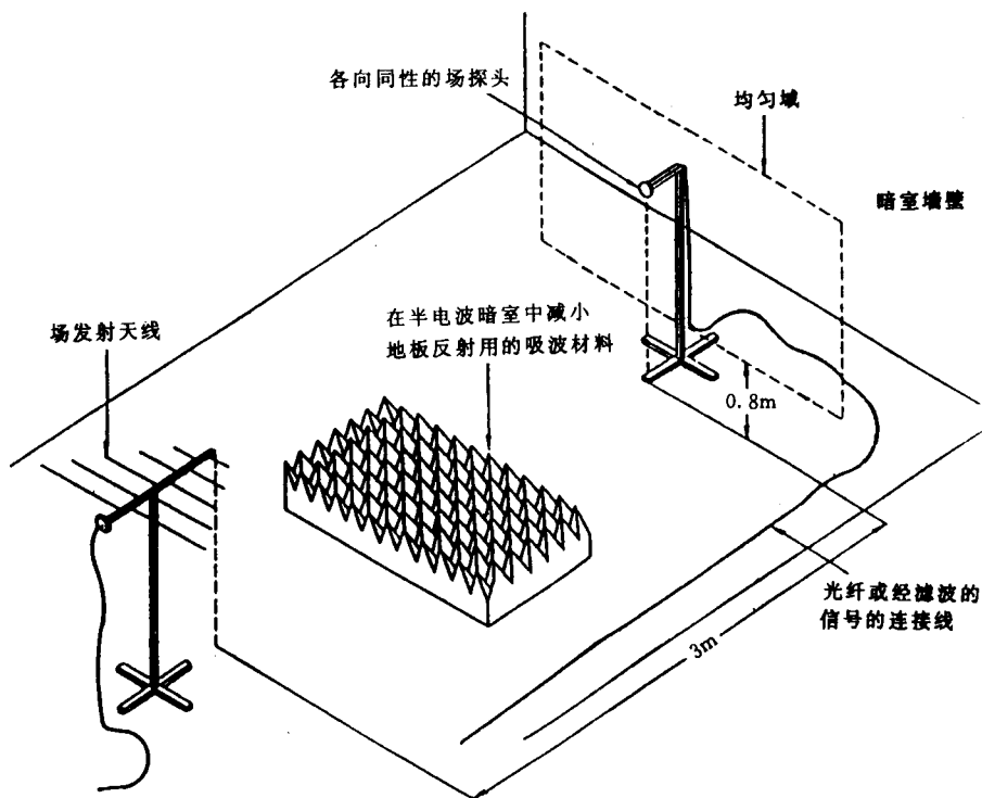
图 3 场校准
