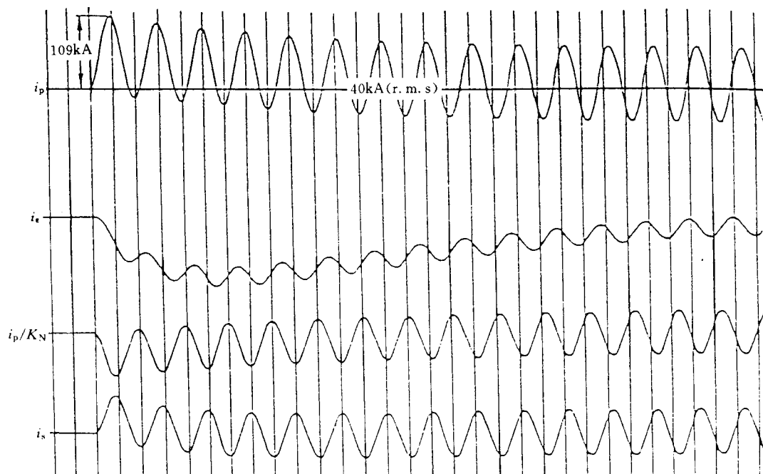
a TPZ 级电流互感器的典型示波图
