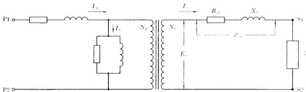
图 E1 电流互感器简化等效电路
