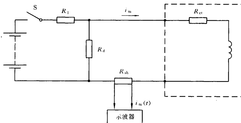
图 B6 另一种直流法电路 1)
