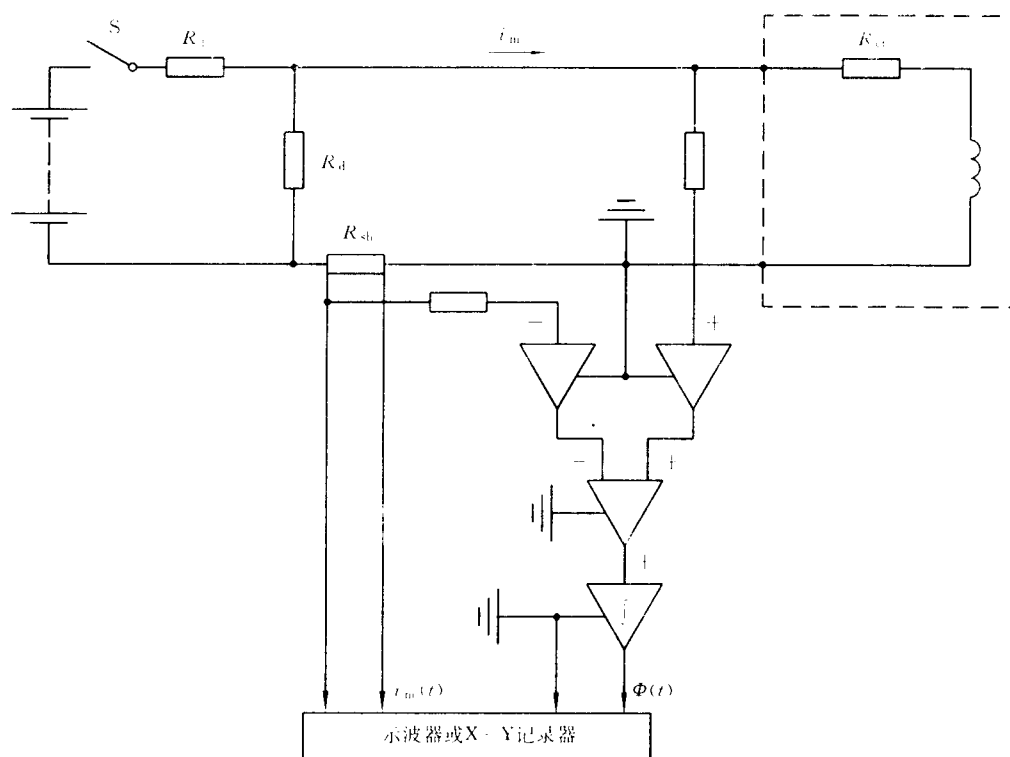
图 B3 直流法基本电路
