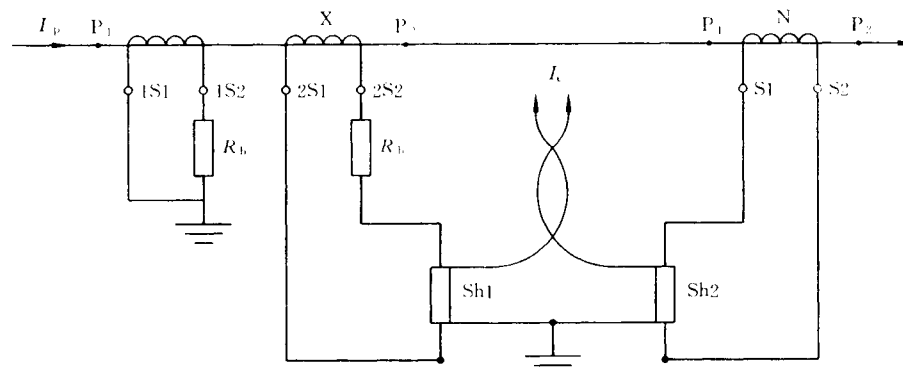
a 采用二次接分流器
