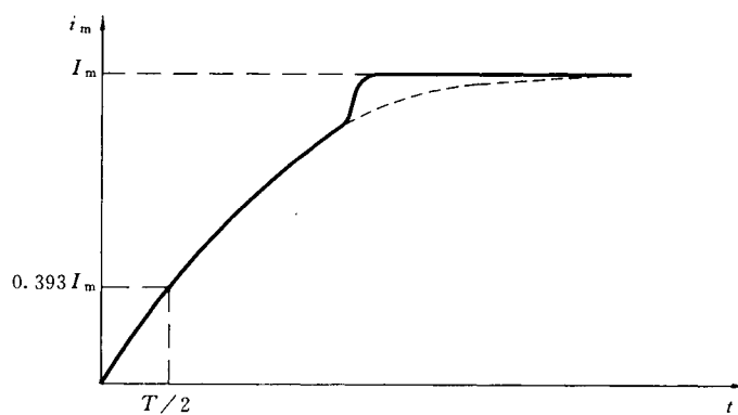
图 B7 另一种直流法的典型记录曲线
