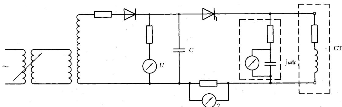
图 B8 电容放电法的电路 1]
