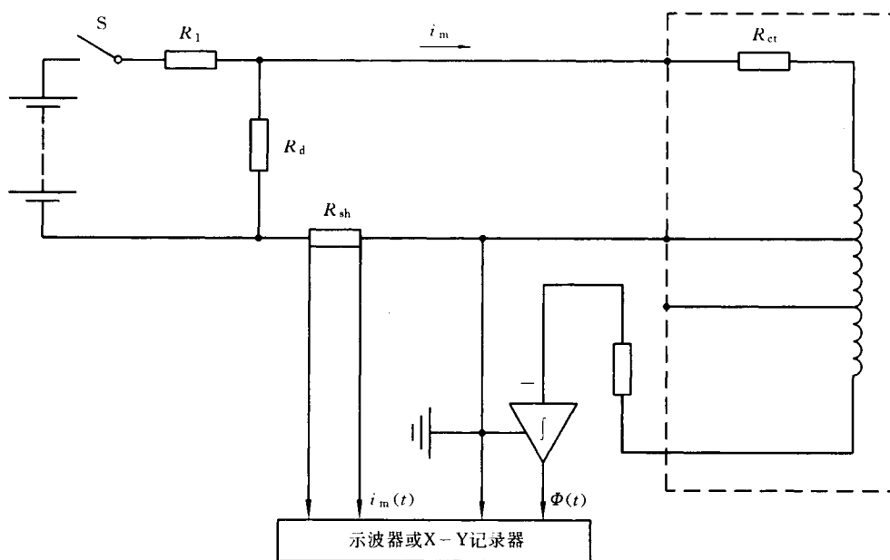
图 B5 用附加的绕组测磁通
