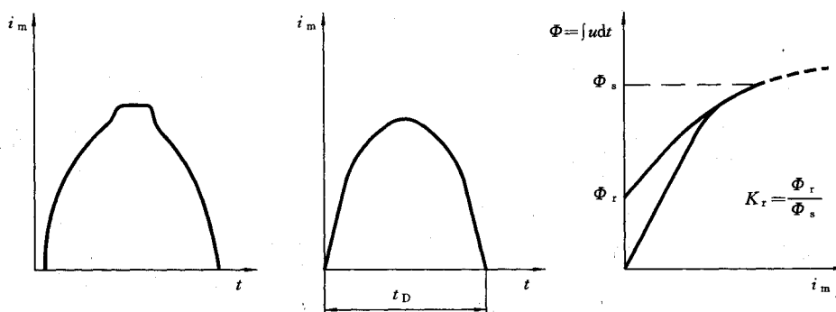
图 B9 电容放电法的典型记录曲线
