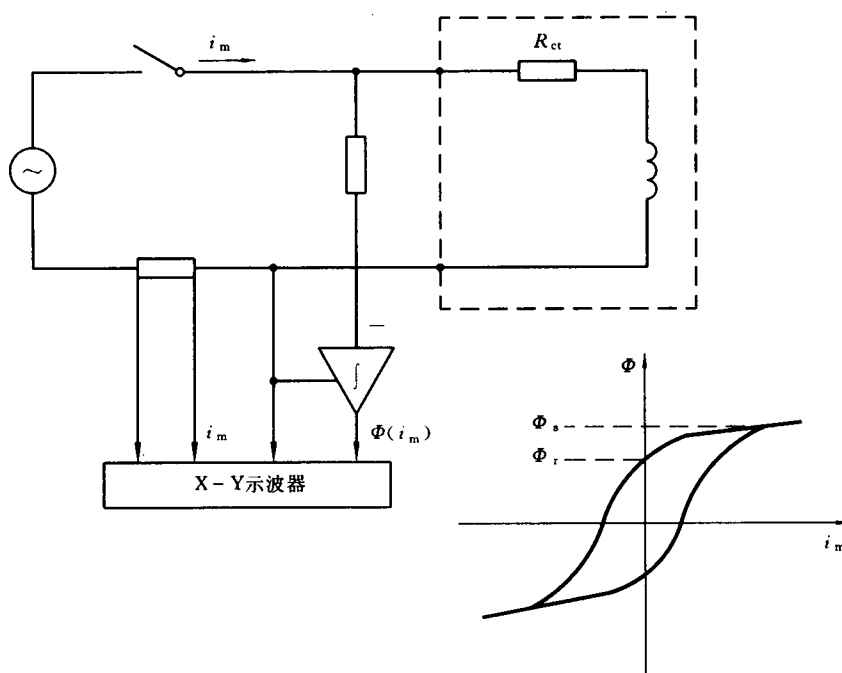
图 B2 用磁滞回环确定剩磁系数 K_r
