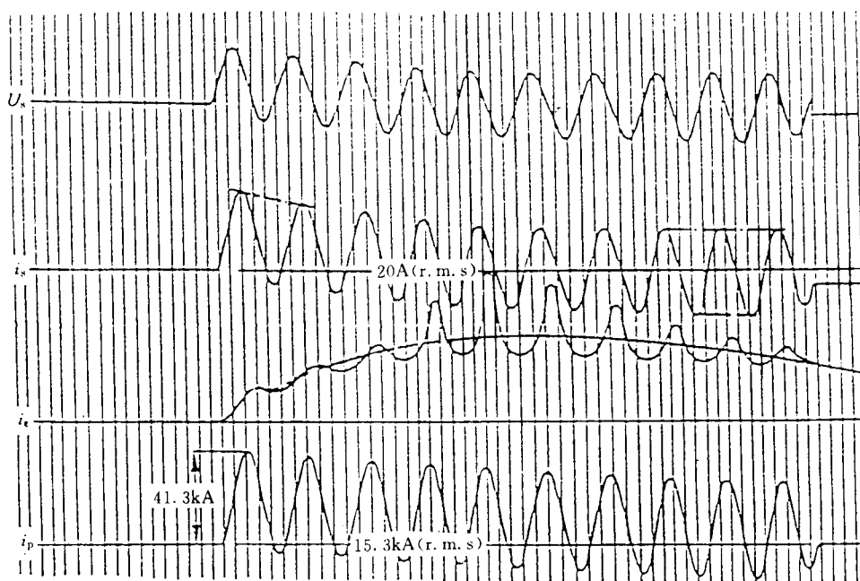
b TPY 级电流互感器的典型示波图
