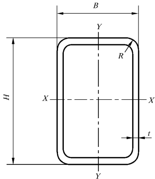
图 2 方形冷弯空心型钢
