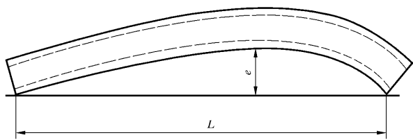
图 6 弯曲度的测定
