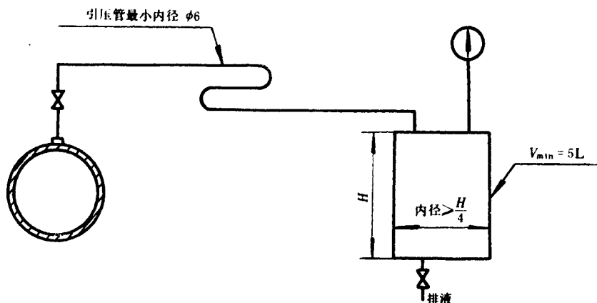
图 7 供测压用的缓冲器示意图
