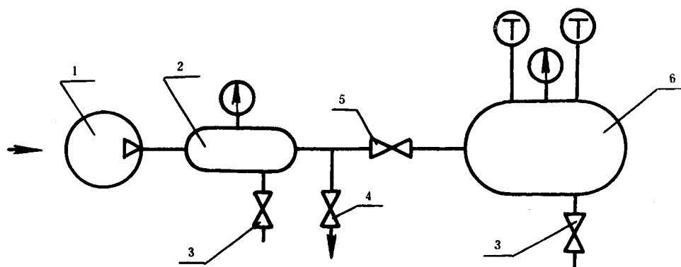
图 A1 充罐法系统示意图
