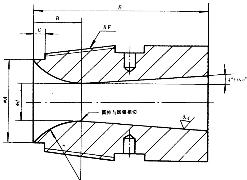
图 12 喷嘴
