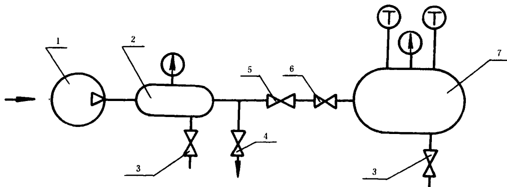
图 B1 称瓶法系统示意图
