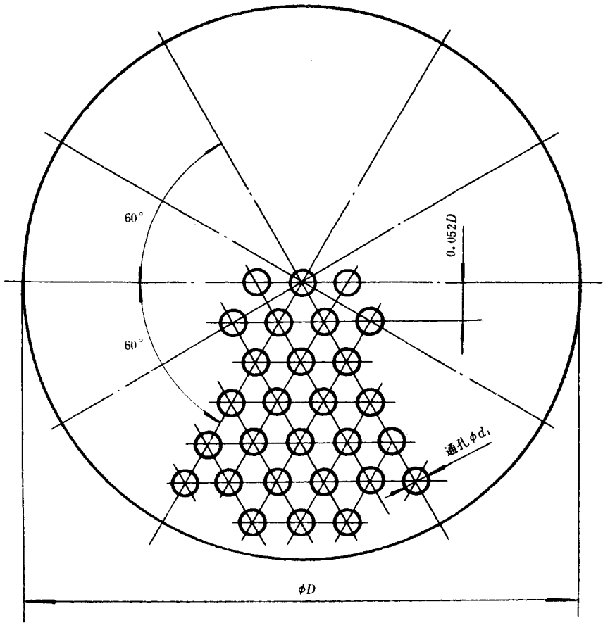
图 6 整流器穿孔板
