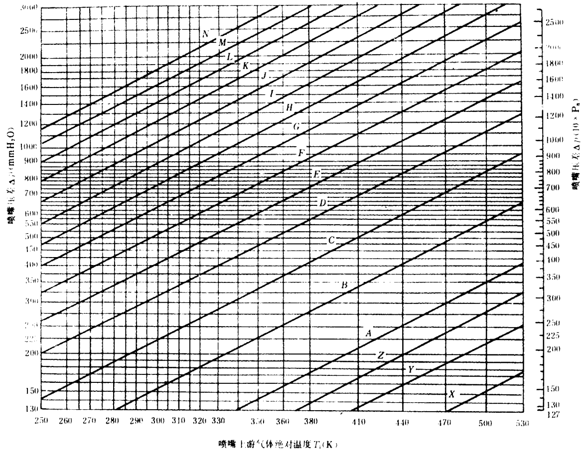
图 10 选择喷嘴系数特性线图
