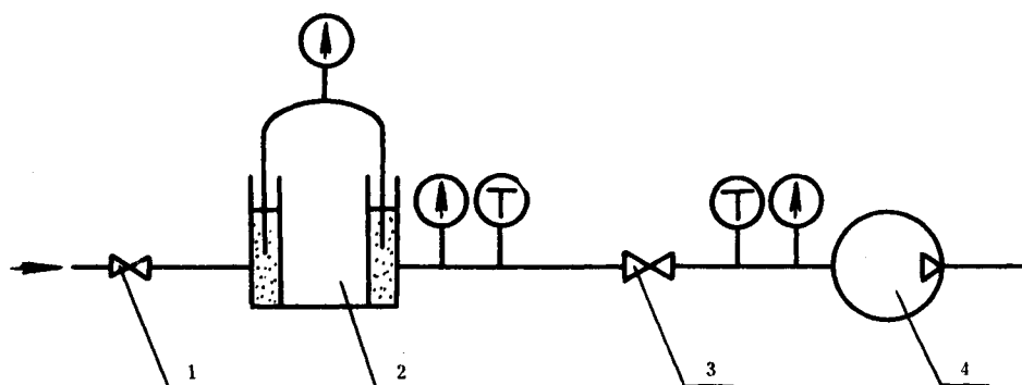
图 C1 气柜法系统示意图
