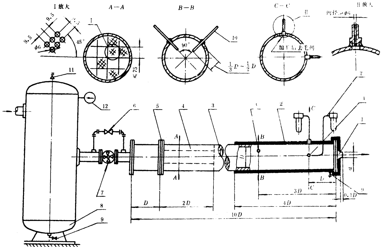
图 8 ASME 喷嘴测量装置示意图
