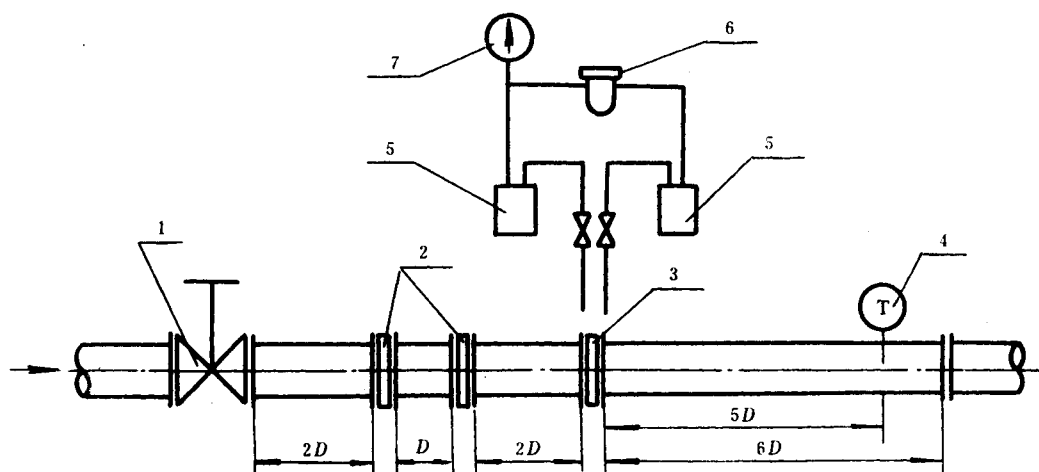
图3 ISA 1932 喷嘴加整流器测量装置示意图
