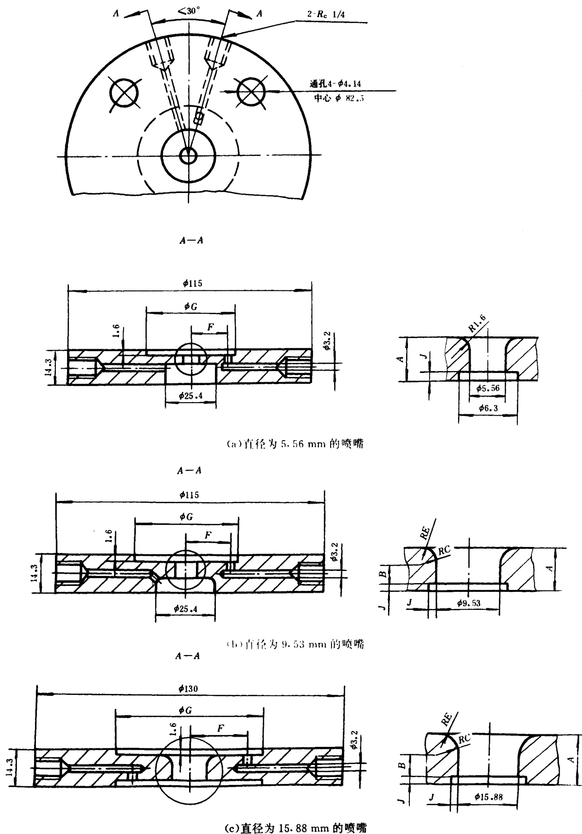
图 4 喷嘴直径 d 不大于 15.88 mm 的喷嘴示意图
