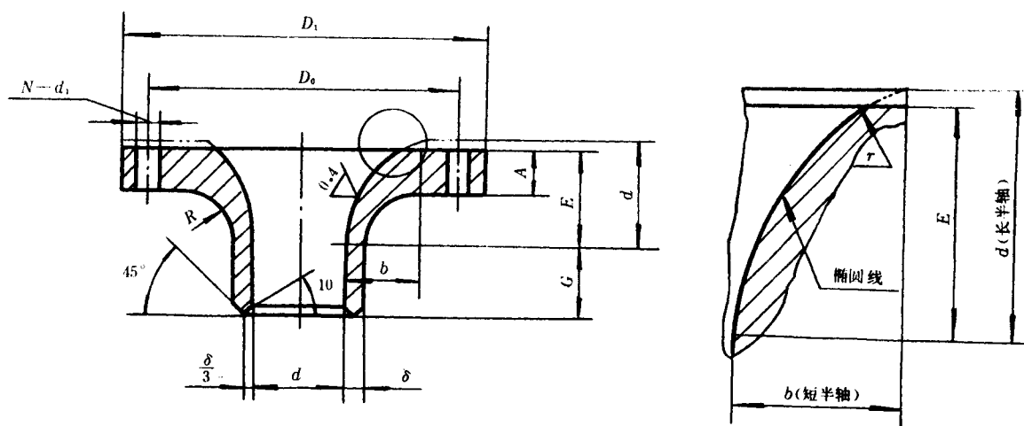
图9 喷嘴
