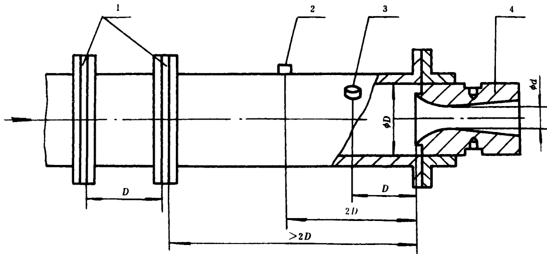
图 11 圆弧文丘里喷嘴测量装置示意图
