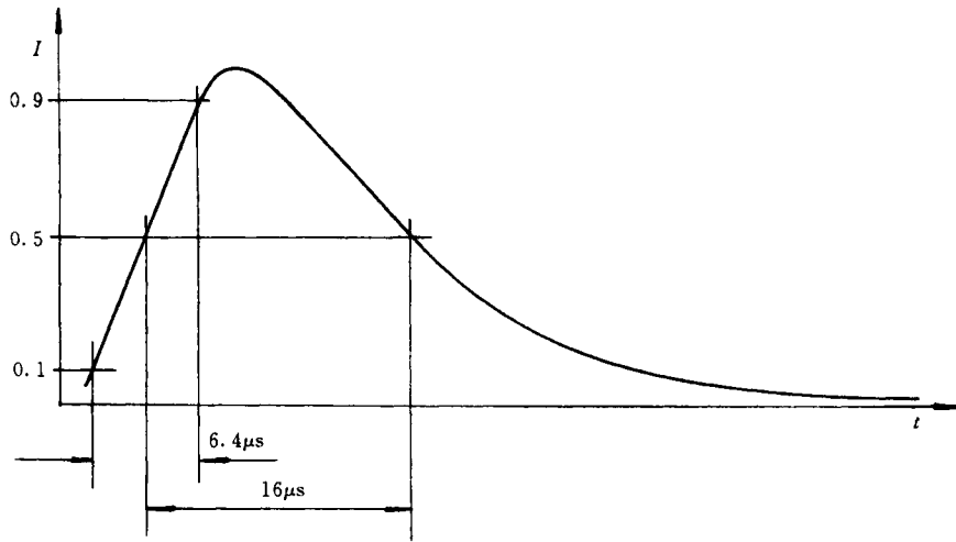
图 2 脉冲磁场试验发生器的输出电流波形(6.4/16 \mu s)
