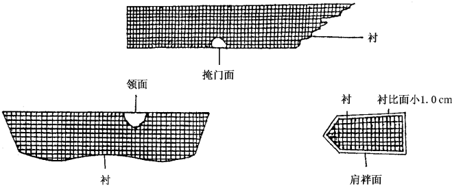
图 4 敷衬工艺
