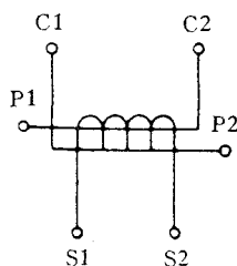
图 8 互感器一次绕组分为两组, 图 9 互感器有两个二次绕组, 各有其铁心(二次绕组有两种标志方法)
