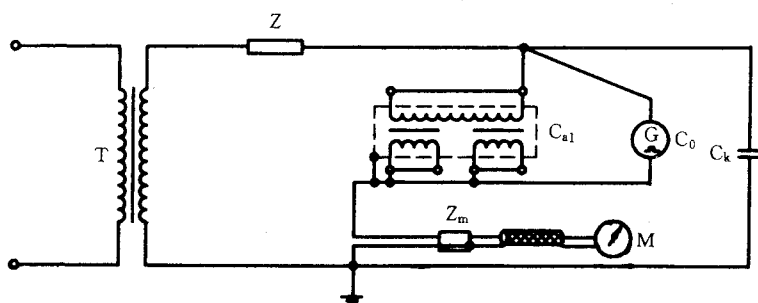
G—带有电容 C_0 的冲击发生器
