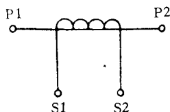
图 6 单电流比互感器
