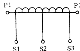
图 7 互感器二次绕组有中间抽头
