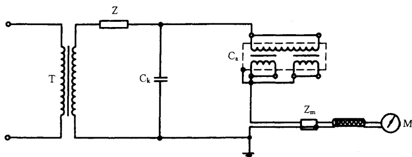
T—试验变压器; C_a —被试互感器; C_k —耦合电容器; M—pD 测量装置; Z_m ——测量阻抗; Z—滤波器(如果 C_k 为试验变压器的电容,则不要求滤波器)
