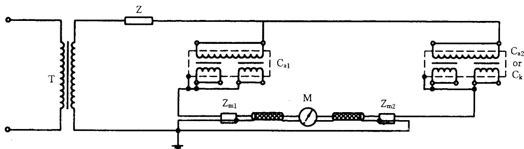
T—试验变压器; C_{a1} —被试互感器; C_{a2} —无局放的试品(或耦合电容器 C_k ); M—局部放电测量仪器; Z_{m1} 、 Z_{m2} ——测量阻抗; Z—滤波器
