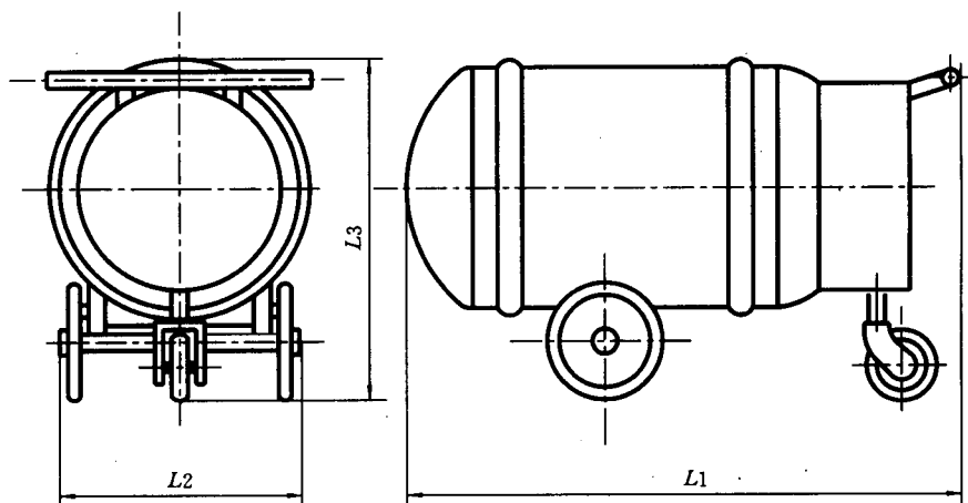
图 2 卧式自增压式液氮容器外形示意图
