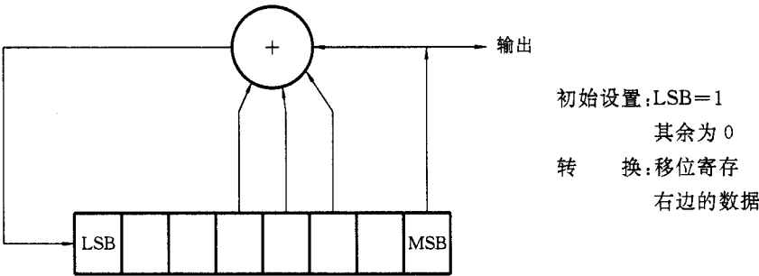
图 11 扰码发生器
