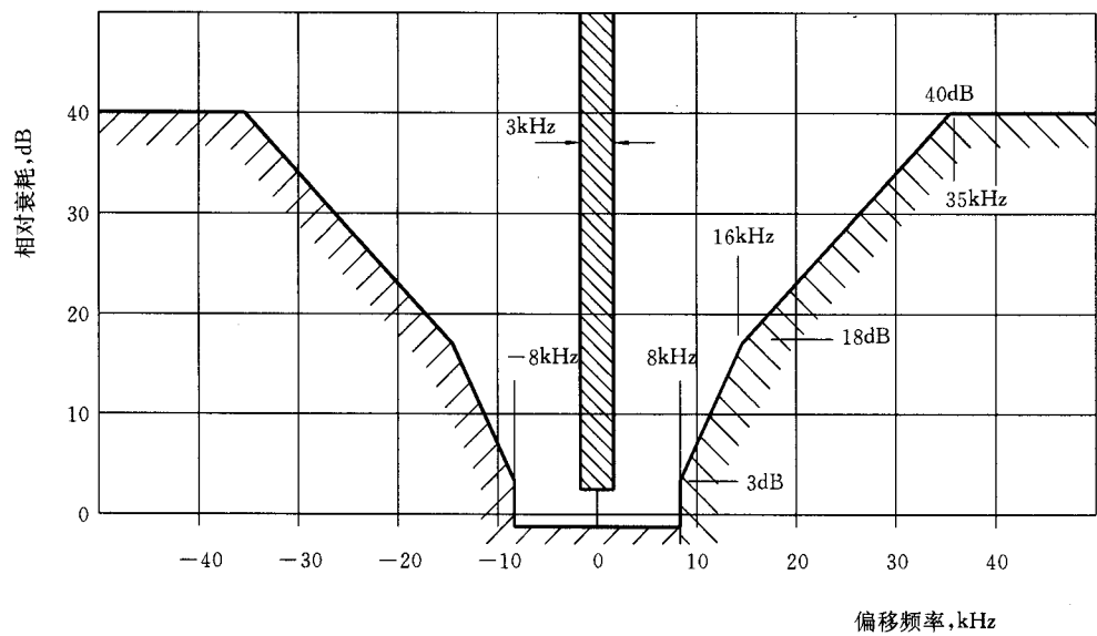
图 12 解调前置滤波器特性
