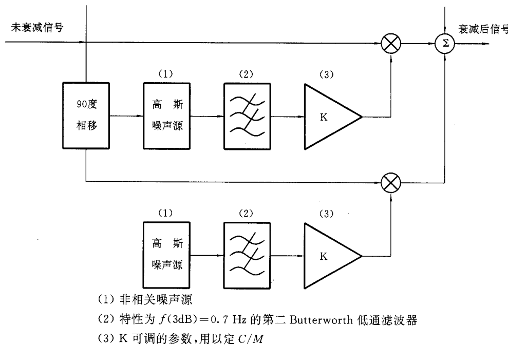
图 13 C 标准离散衰减分布框图
