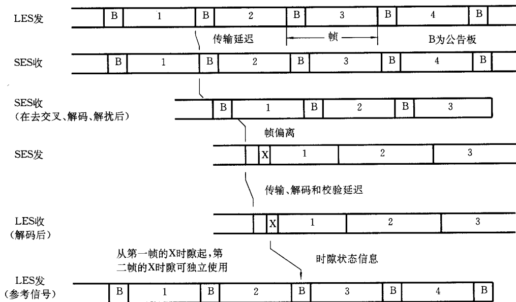
图 14 2 帧时隙的传送过程
