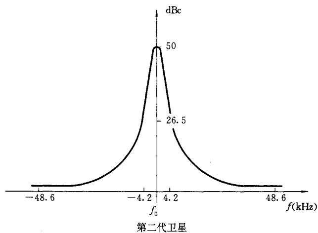
图 4 发射频谱
