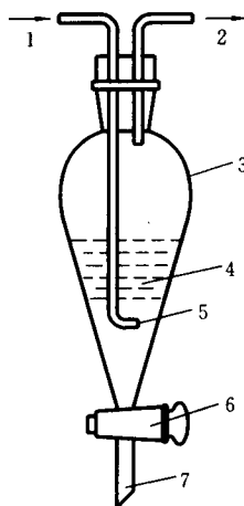
1—气体进口;2—气体出口;3—分液漏斗(500 mL);4—试油; 5—散气元件(具微孔烧结板);6—旋塞;7—油出口
