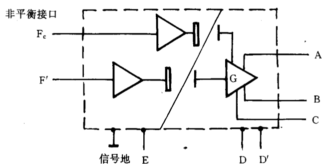
A, B—平衡信号输出; C—零电压参考互换点; D, D'—浮地电源; E—非平衡站电源; F'—非平衡信号输入; Fc—非平衡高阻抗控制; G—隔离的发生器
