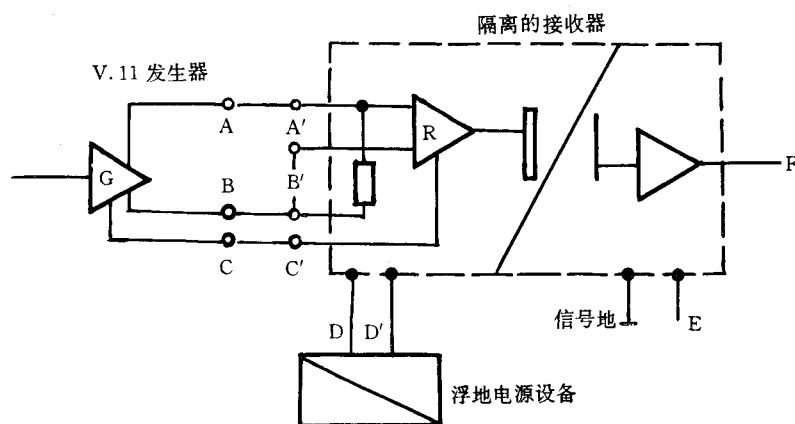
图 A2 GB 7619 发生器与隔离的接收器的互连
