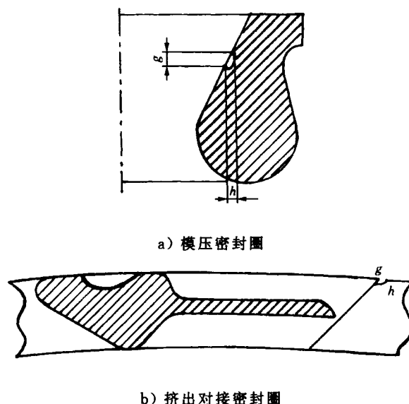
图 4 开模缩裂和分模线凹陷
