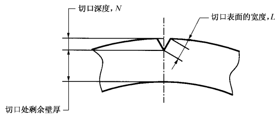
图 3 切口几何尺寸示意图
