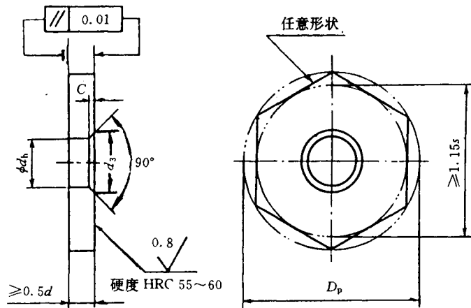
d —螺纹公称直径; s —螺栓、螺母对边宽度; D_p —垫片的最大直径或外接圆直径; d_h —接触的支承面内径(GB 5277, 中等装配系列); d_3 —按 GB 152.4 的规定
