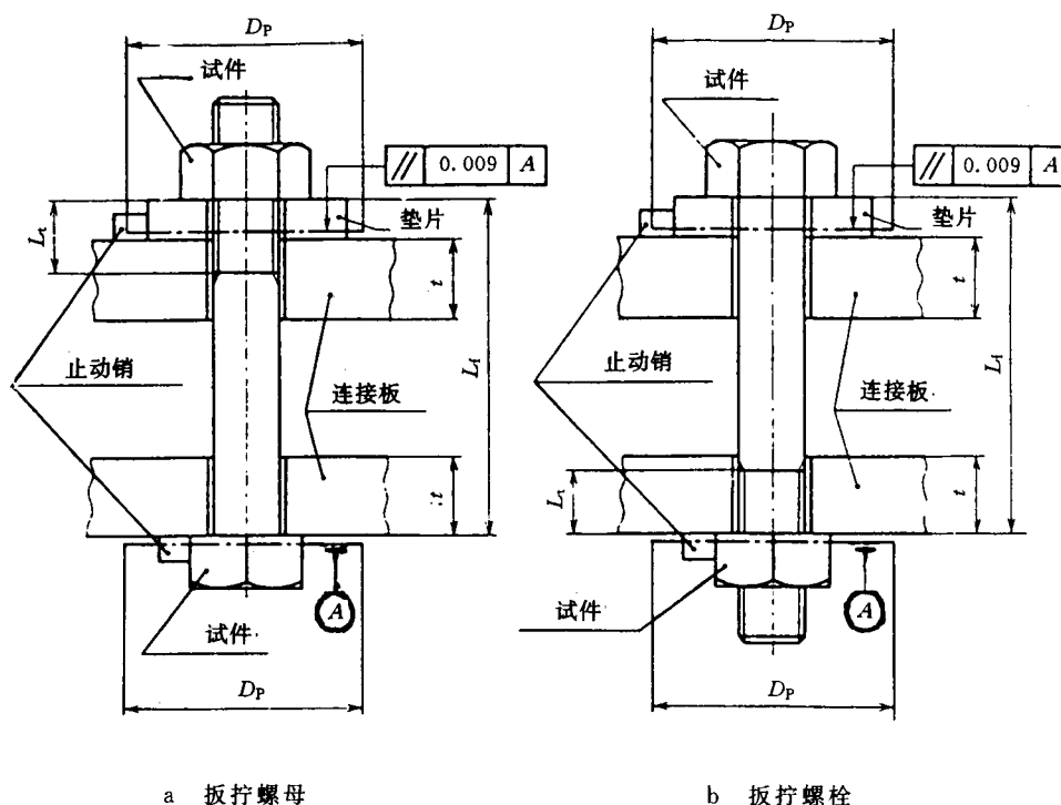
a 板拧螺母 b 板拧螺栓 D_p —垫片的最大直径或外接圆直径,见图2; L_t —螺栓支承面与螺母支承面间的距离; L_t —螺栓、螺母支承面间的螺纹长度, L_t \geq 6P ( P —螺距); t \geq d ( d —螺纹公称直径)
