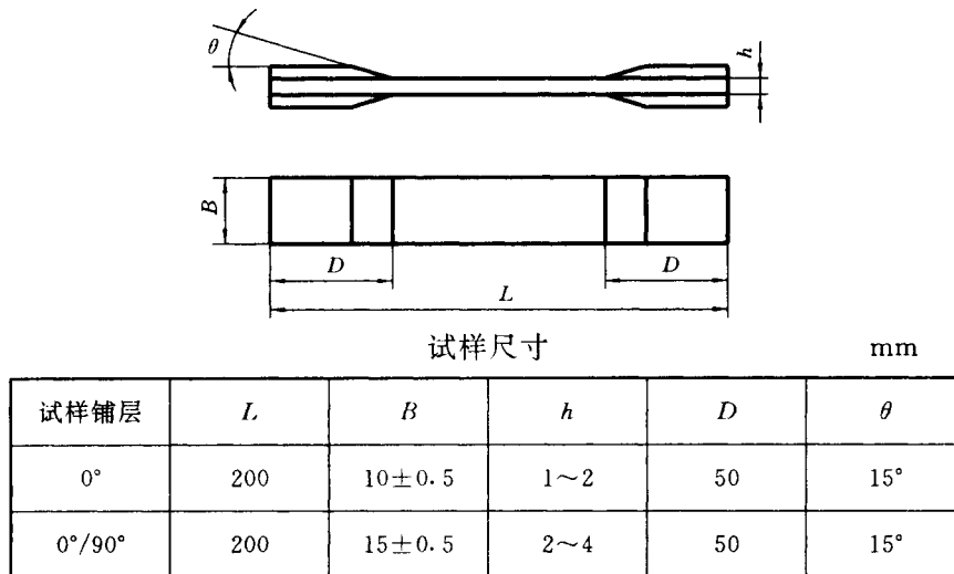
图 2 直条试样
