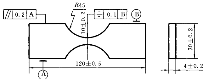
图 3 哑铃形试样
