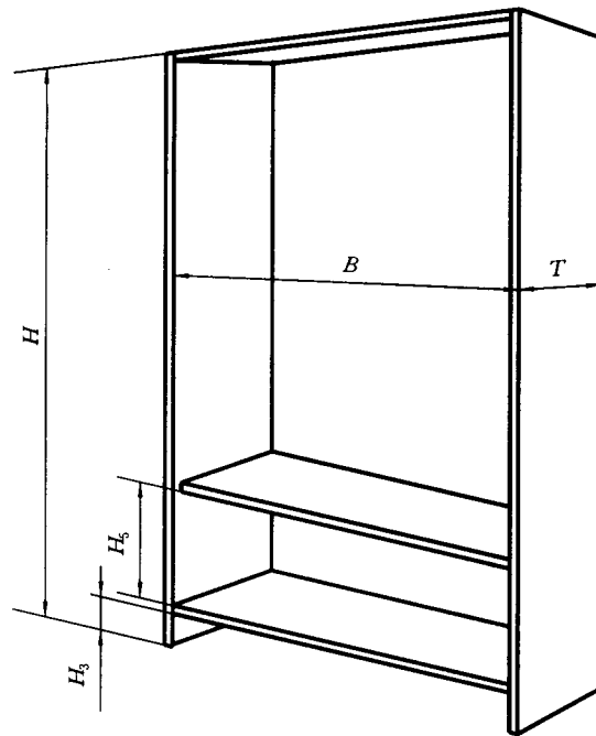
图 4 书柜尺寸示意图
