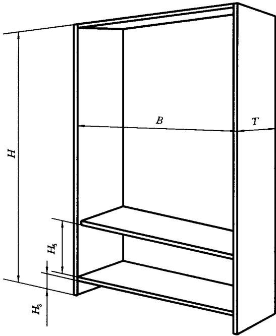
图 5 文件柜尺寸示意图
