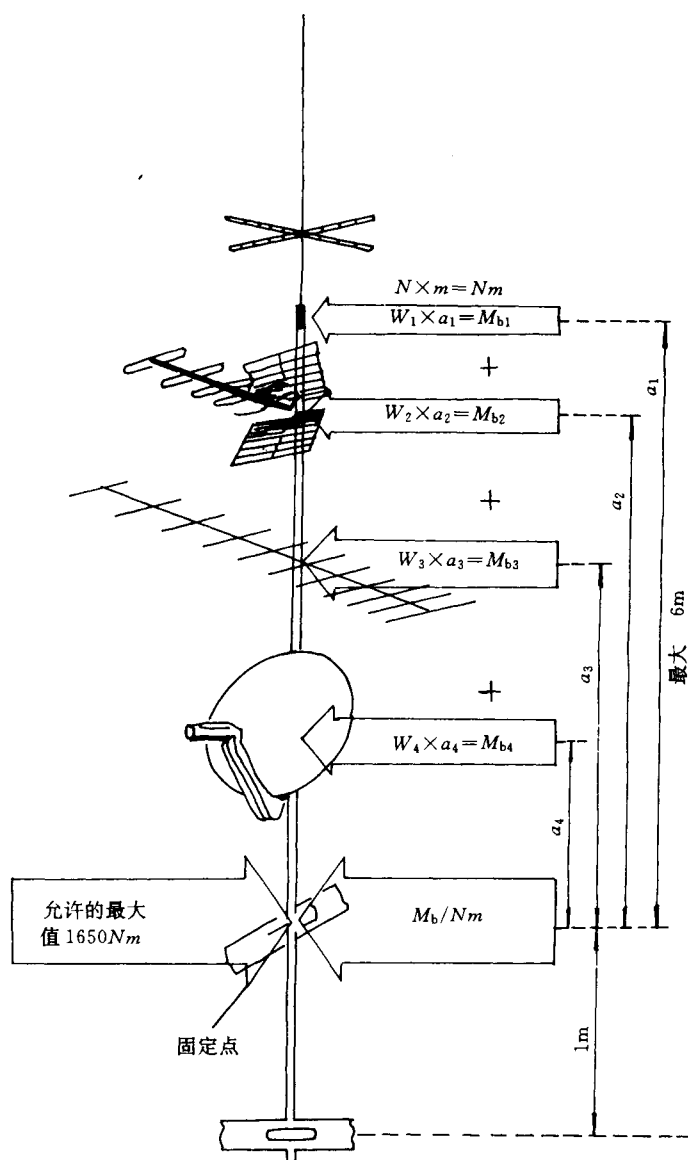
图 40 天线杆的弯曲力矩
