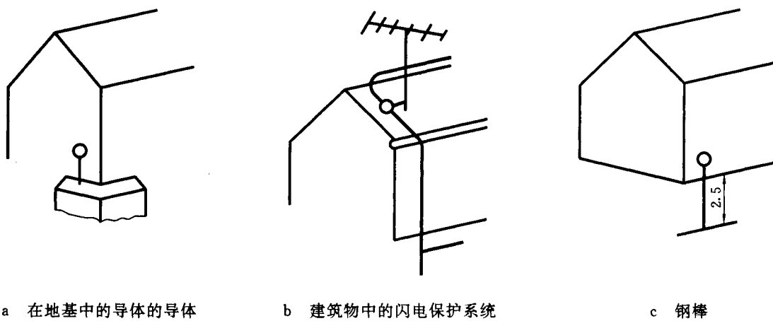
图 39 接地机构的例子
