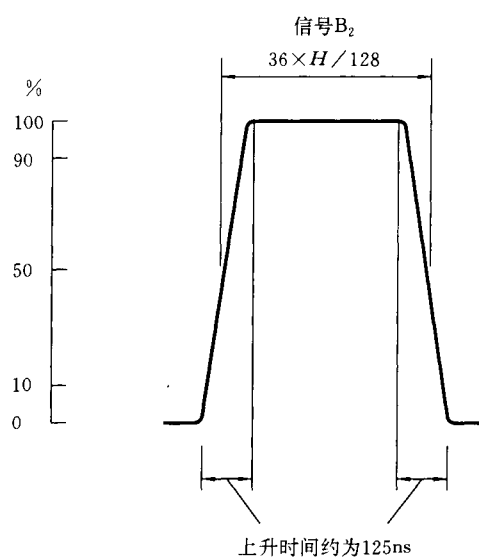
b 525 行制式的信号 B
