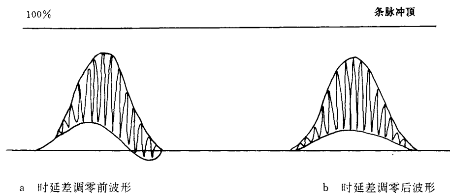
图 7 显示脉冲:色度信号低且滞后
