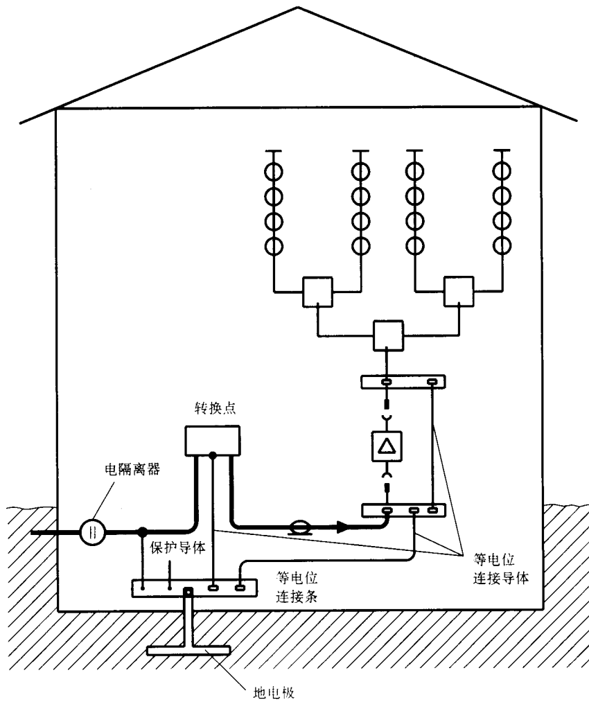
图 35 等电位连接电隔离的电缆进入建筑物的例子(地下连接)
