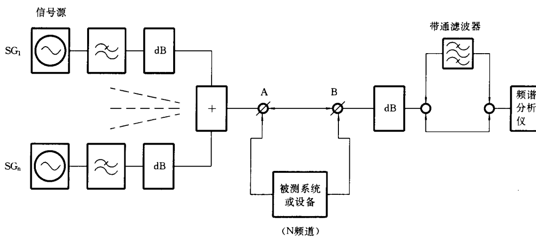
图 11 用组合差拍测量非线性失真测试的设备连接
