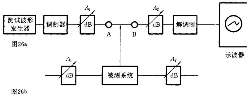
图 26 回波值测量的测试设备的布置
