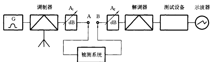
图 6 色度/亮度增益和时延差测量的设备连接
