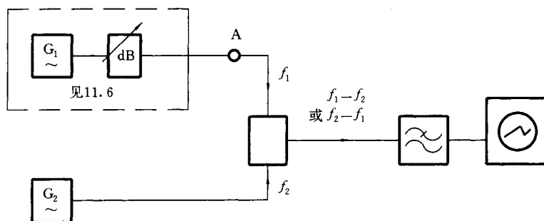
图 G1 调制度的校准
