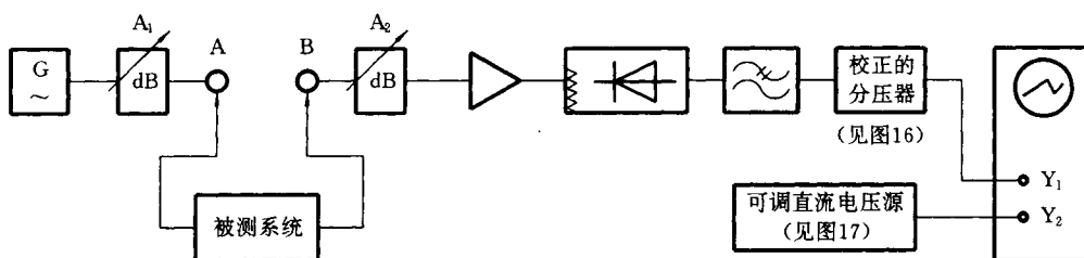
图 15 交流声调制测量的设备连接(直流法)
