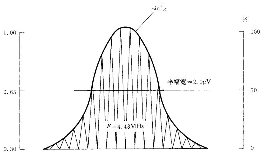
图 4 用于色度/亮度增益和时延差的测试信号
