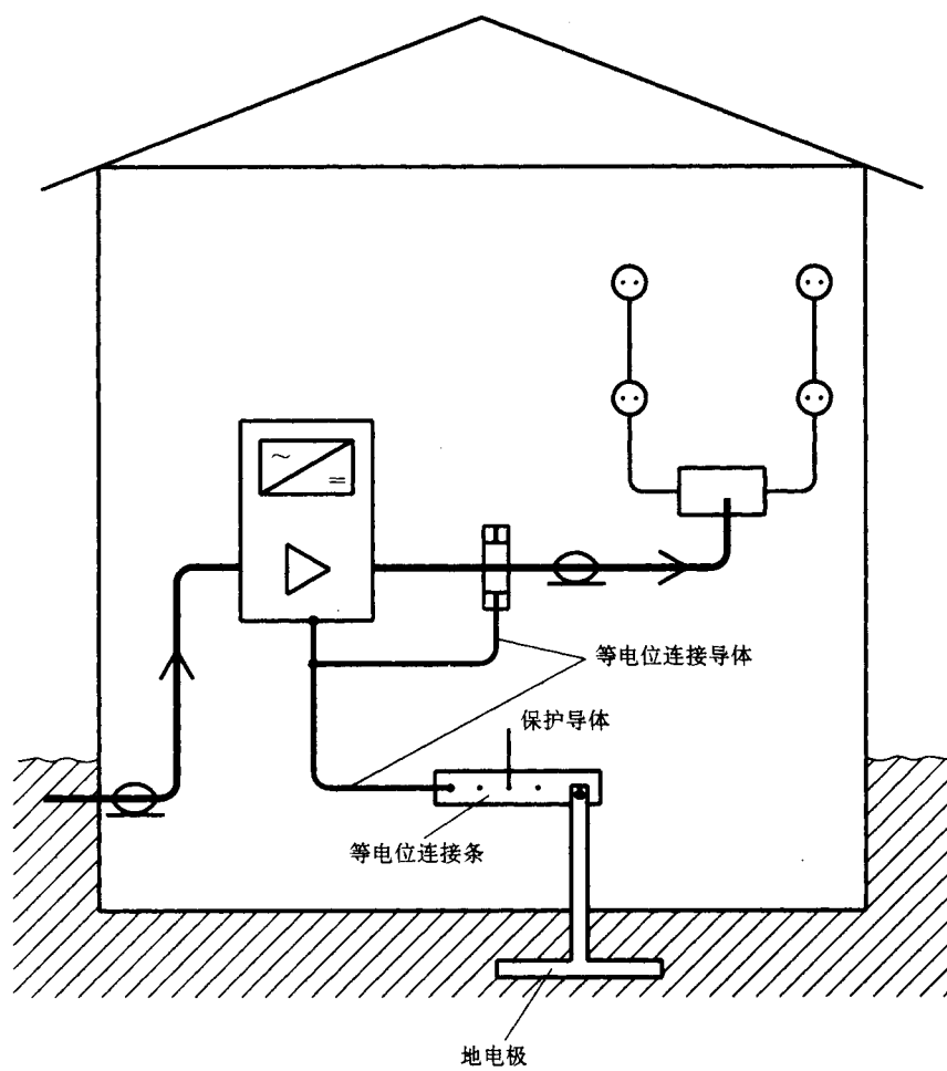
图 37 外部安全等电位连接的例子
