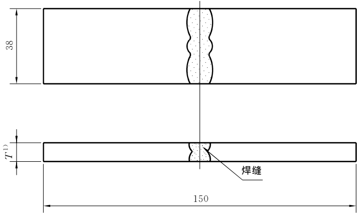
图 6 弯曲试验用试样
