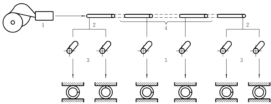
1—焊接;2—钢带端头;3—切端头,2个试样; 4—焊接停止;5—2个试样,焊接停止时两端各取1个
