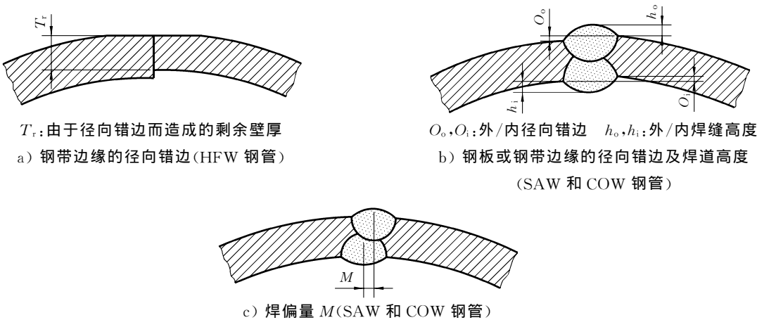
图 2 可能的焊缝尺寸偏差
