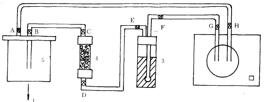
测定系统图
