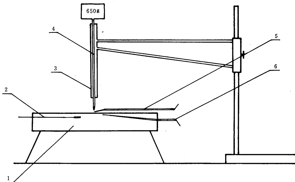
图 B1 表面温度的测量
