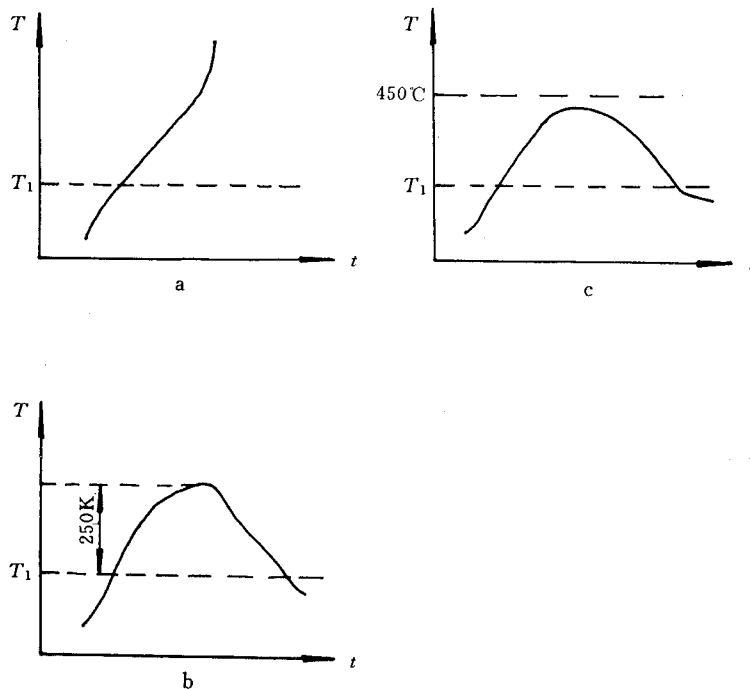
图 3 热表面上粉尘层的典型温度时间曲线
