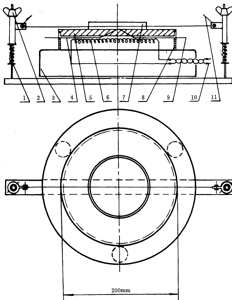
图 1 试验装置示意图
