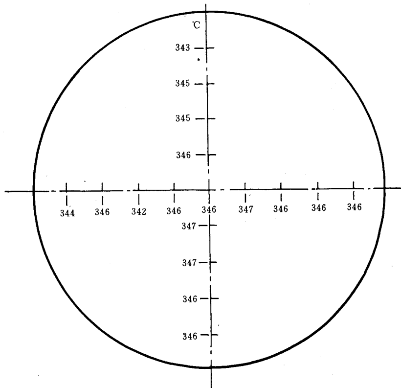
图 B2 典型表面温度分布
