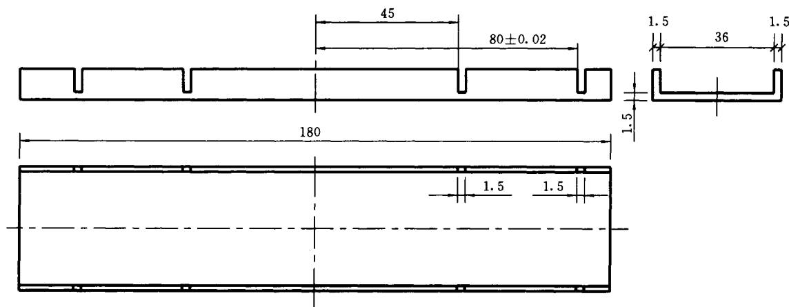
图4 不锈钢槽板
