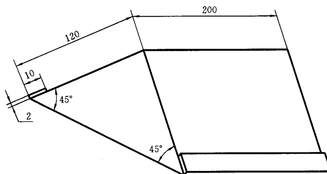
图 1 试样架
