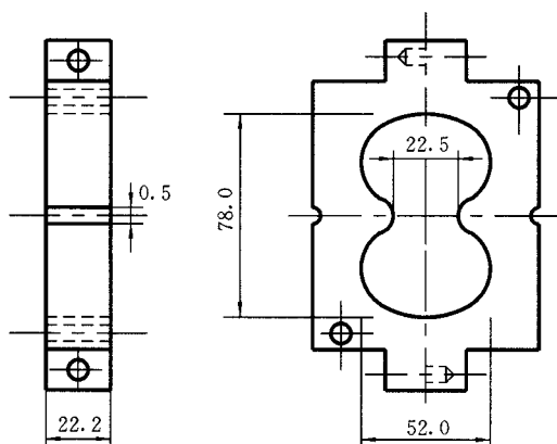
图 2 “8”字形金属模具
