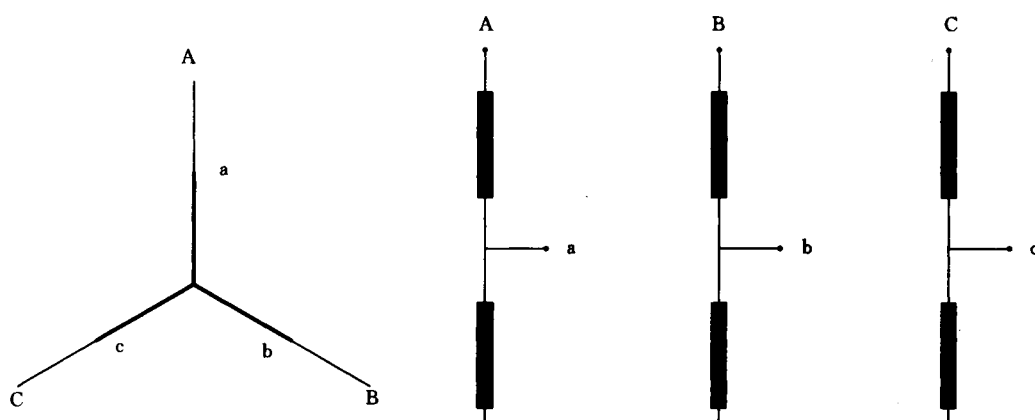
图 D3 三相自耦变压器联结组举例 (联结组标号 Yd0)
