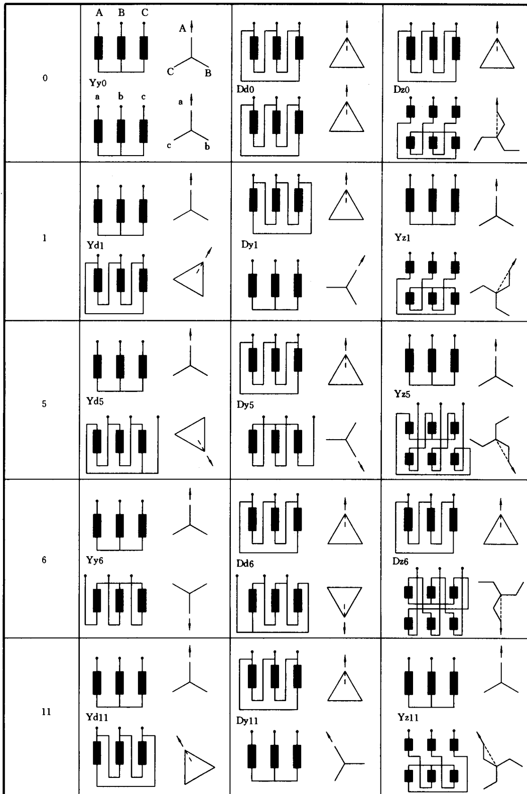
图 D1 常用的联结组
