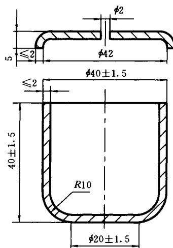
图 3 坩埚和盖
