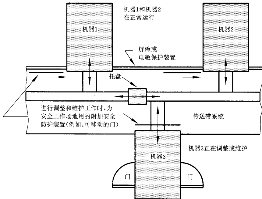
图 A3 调整和维护用的附加安全措施示例
