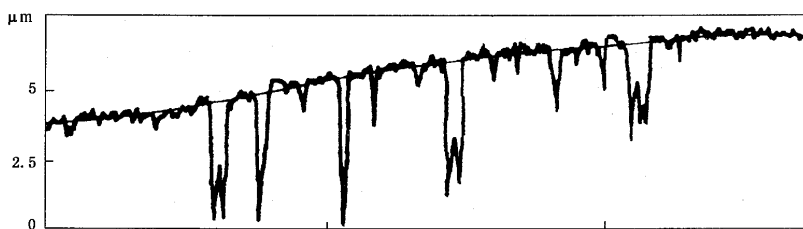
c) 基础线在消除谷后且未滤波的原始轮廓上的位置
